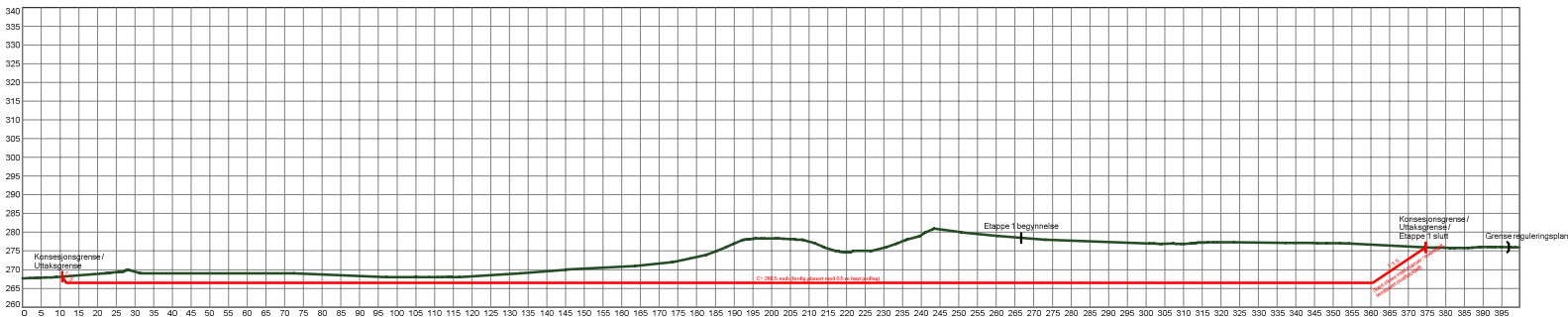
Avslutningsplan (lengdeprofil)
