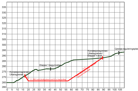
Avslutningsplan (tverrprofil)
