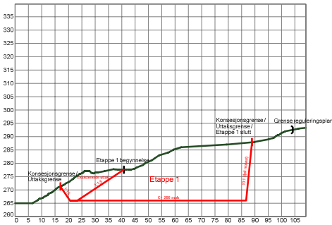
Eksisterende uttak og etappe 1 (tverrprofil)
