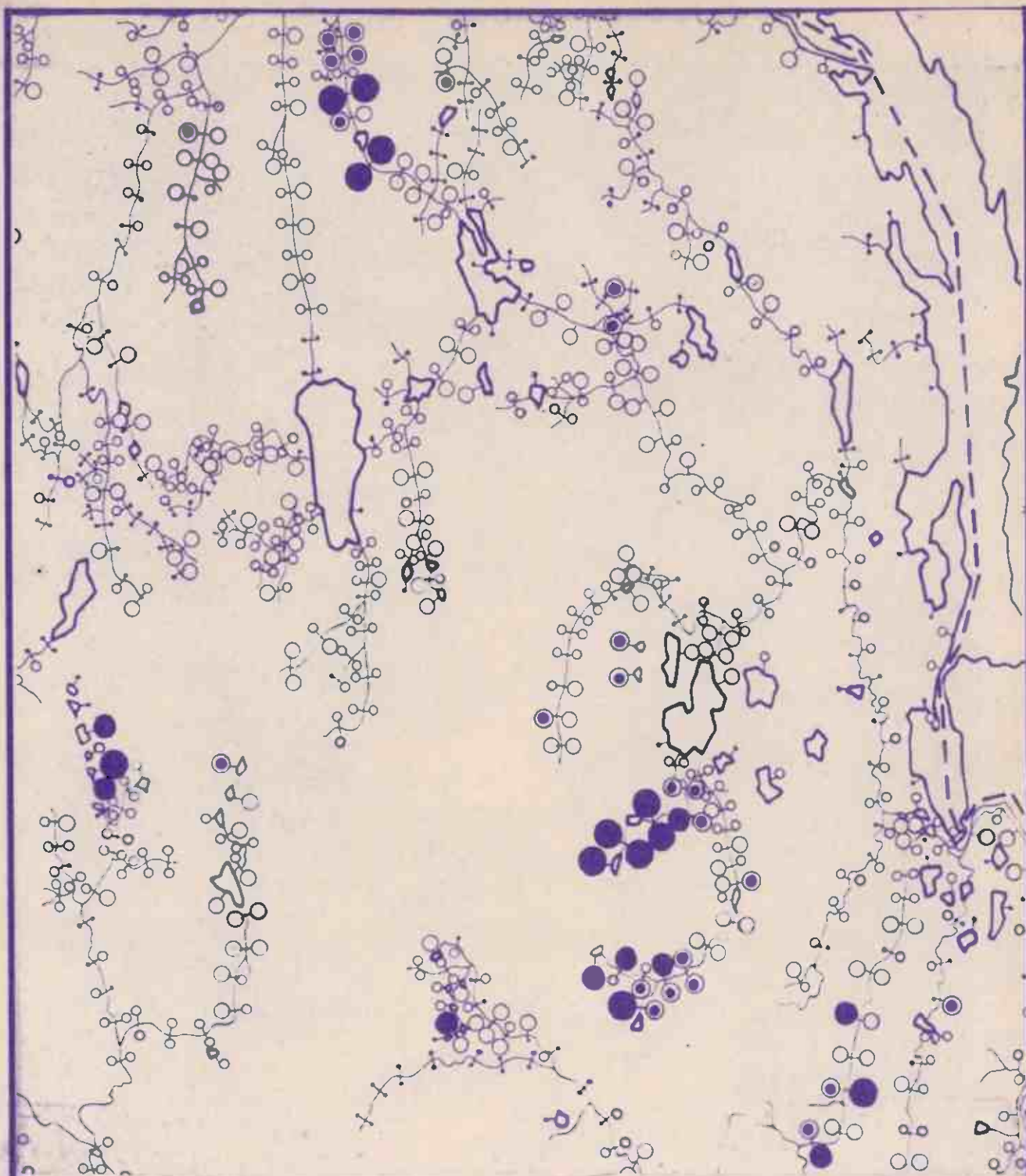
Geokjemiske anomalier (Cu) i bekkesedimenter (for tegnforklaring se Pl. 16)
