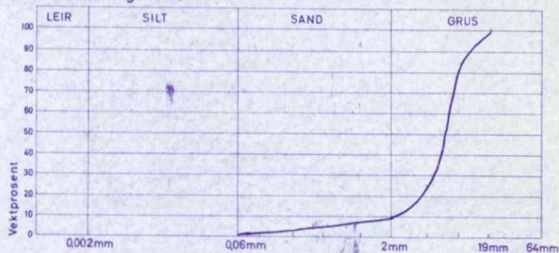
Kornfordelingskurve
