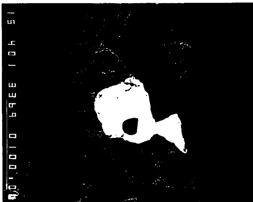
Figur 11. BSE-bilde av sonerte nikkel-mineraler. Innerst milleritt, deretter en rand med gersdorffitt og ytterst pentlanditt sammenvokst med noe magnetkis. Til høyre sonerte krom-spineller. Strek til venstre er 0.1 mm.
