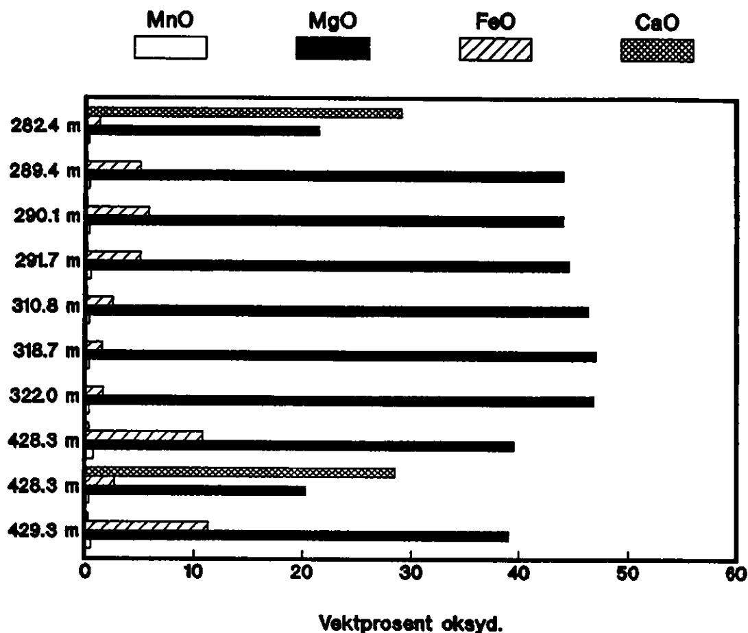
Figur 3. Variasjon i karbonatenes kjemi over et tverrsnitt av den ultramafiske kroppen. Søylenes representerer gjennomsnittet av analysene for den dominerende karbonat-typen ved det aktuelle dyp. Avstanden mellom prøvene er ikke konstant.
