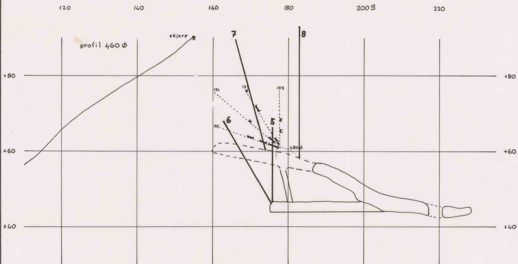
mojell Grube, linse I nord. Forslag diamantboring
