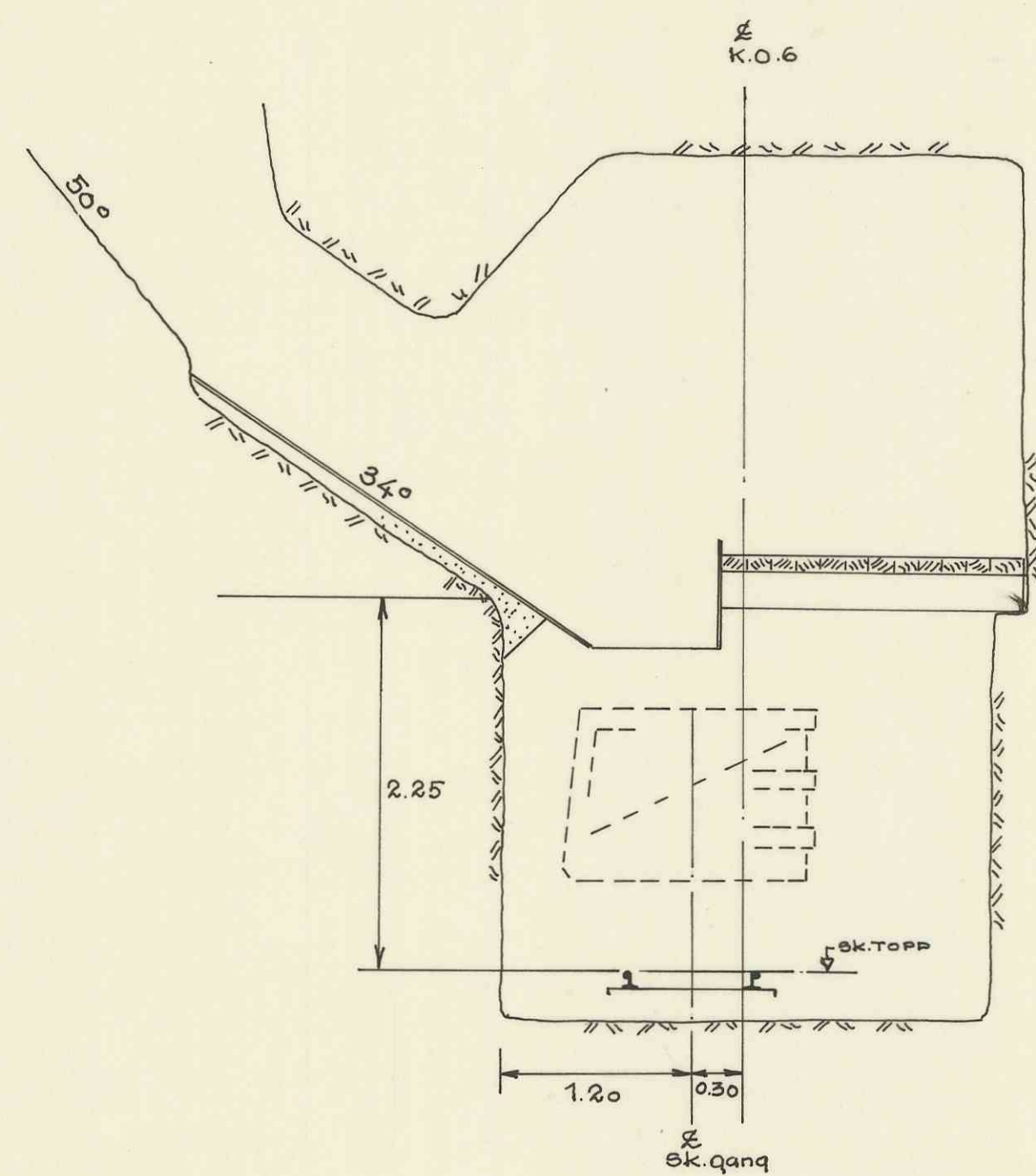
SNITT A-A M. 1:40
