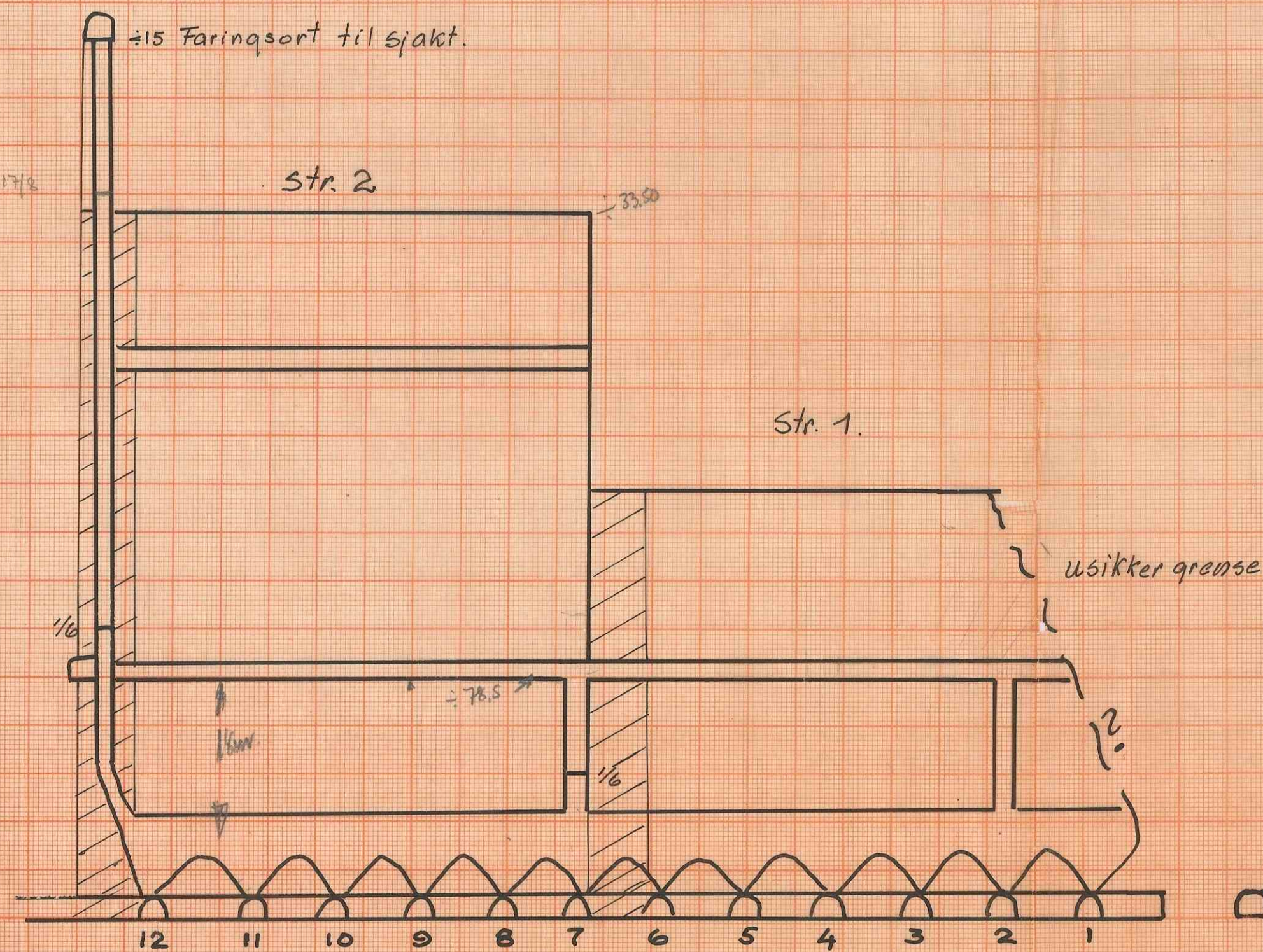
Lengdesnitt gjennom str. log 2 i C IV b . stiqorter og mellomorter.
