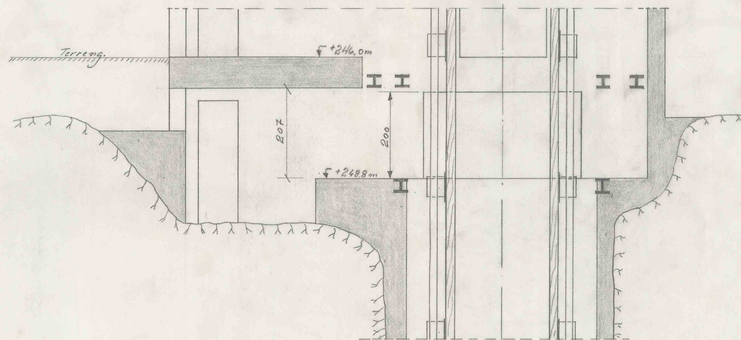
SNITT B-B.
