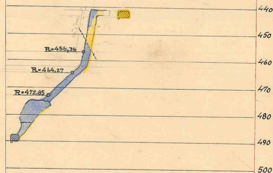
Tverprofil fra stigort ~ 30 m vest prf 22
