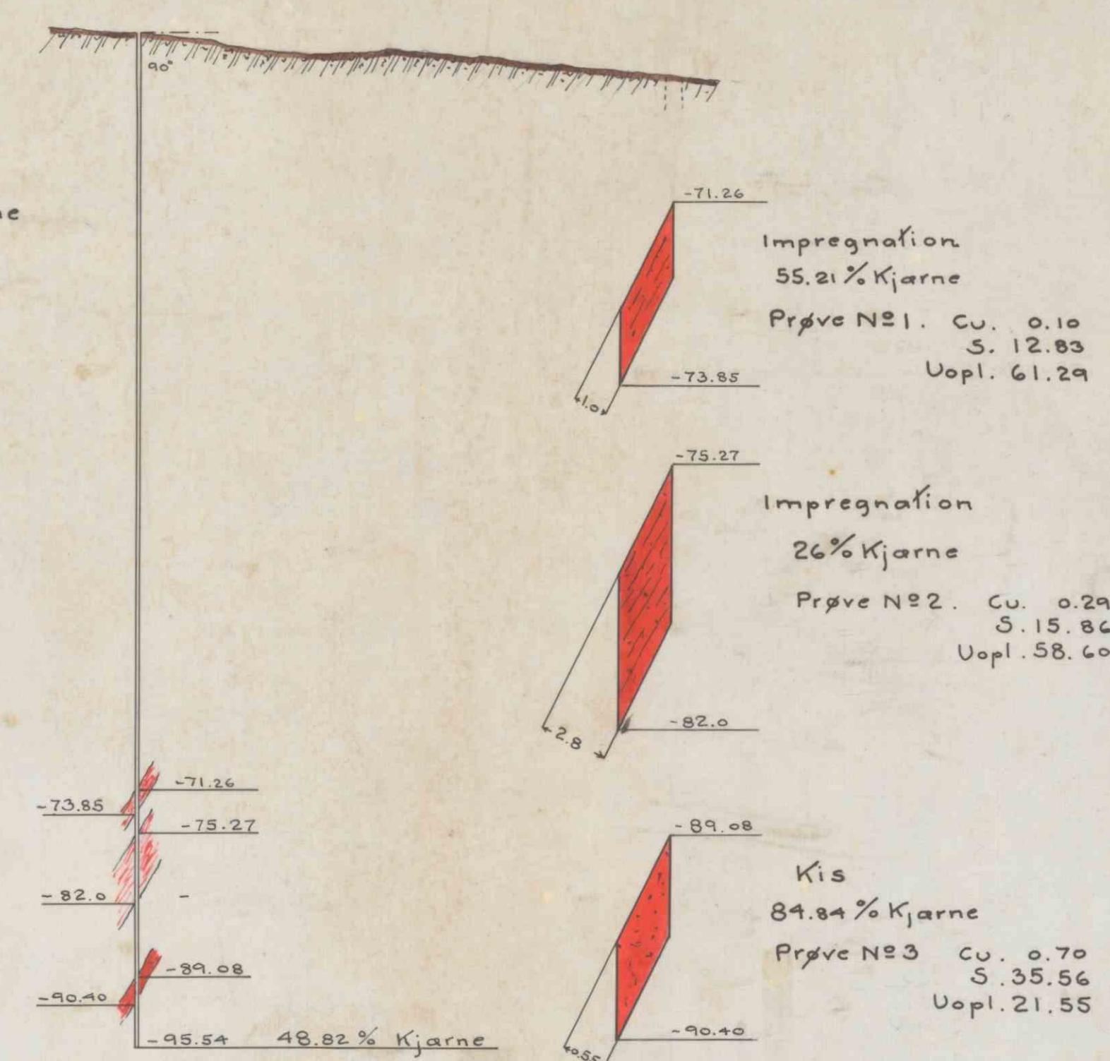
Borhul Nº8 1:500
