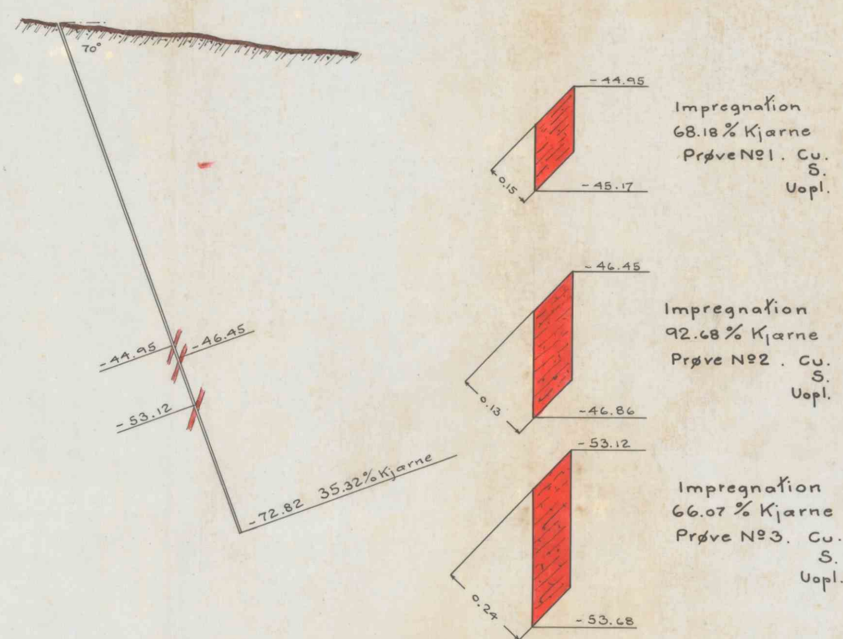
Borhul Nº6 1:500
