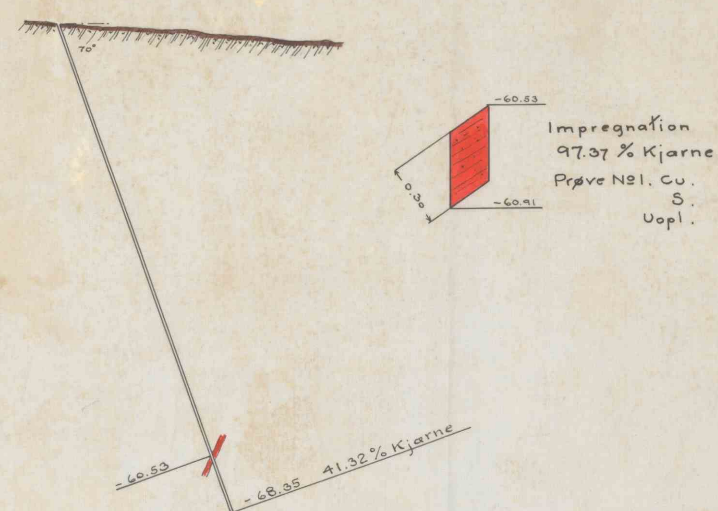
Borhul Nº7 1:500
