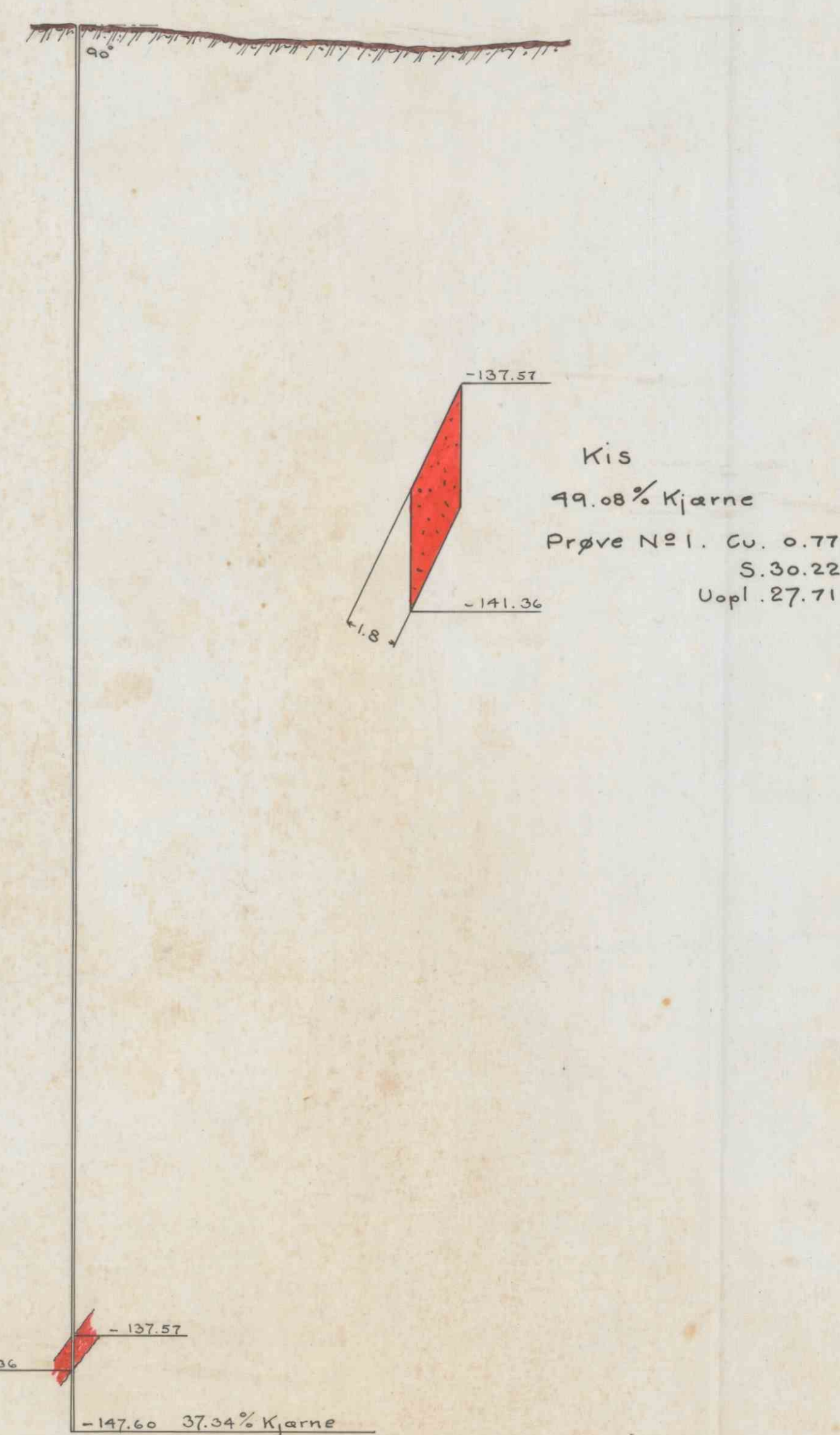
Borhul Nº11 1:500
