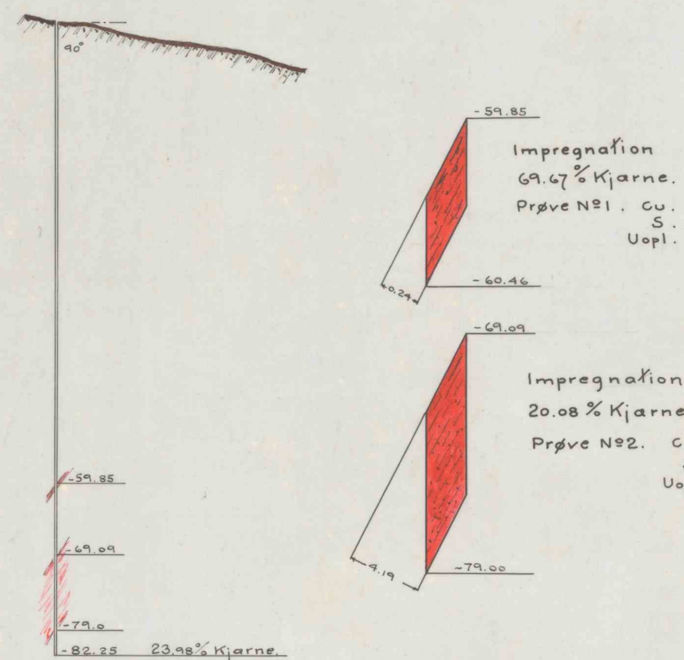
Borhul Nº5 1:500
