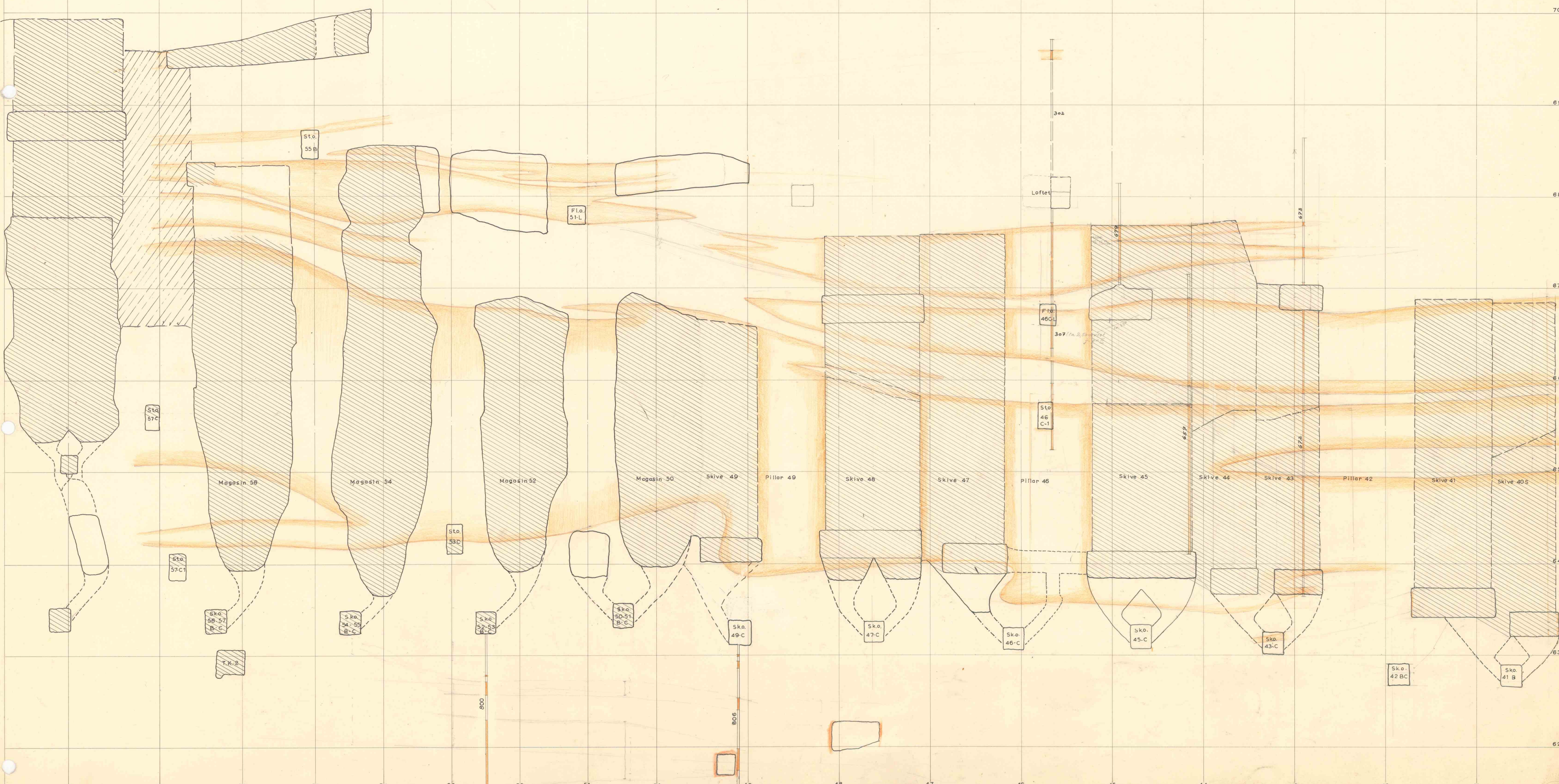
Profil II - s 41-58 M. 1:200 13142
