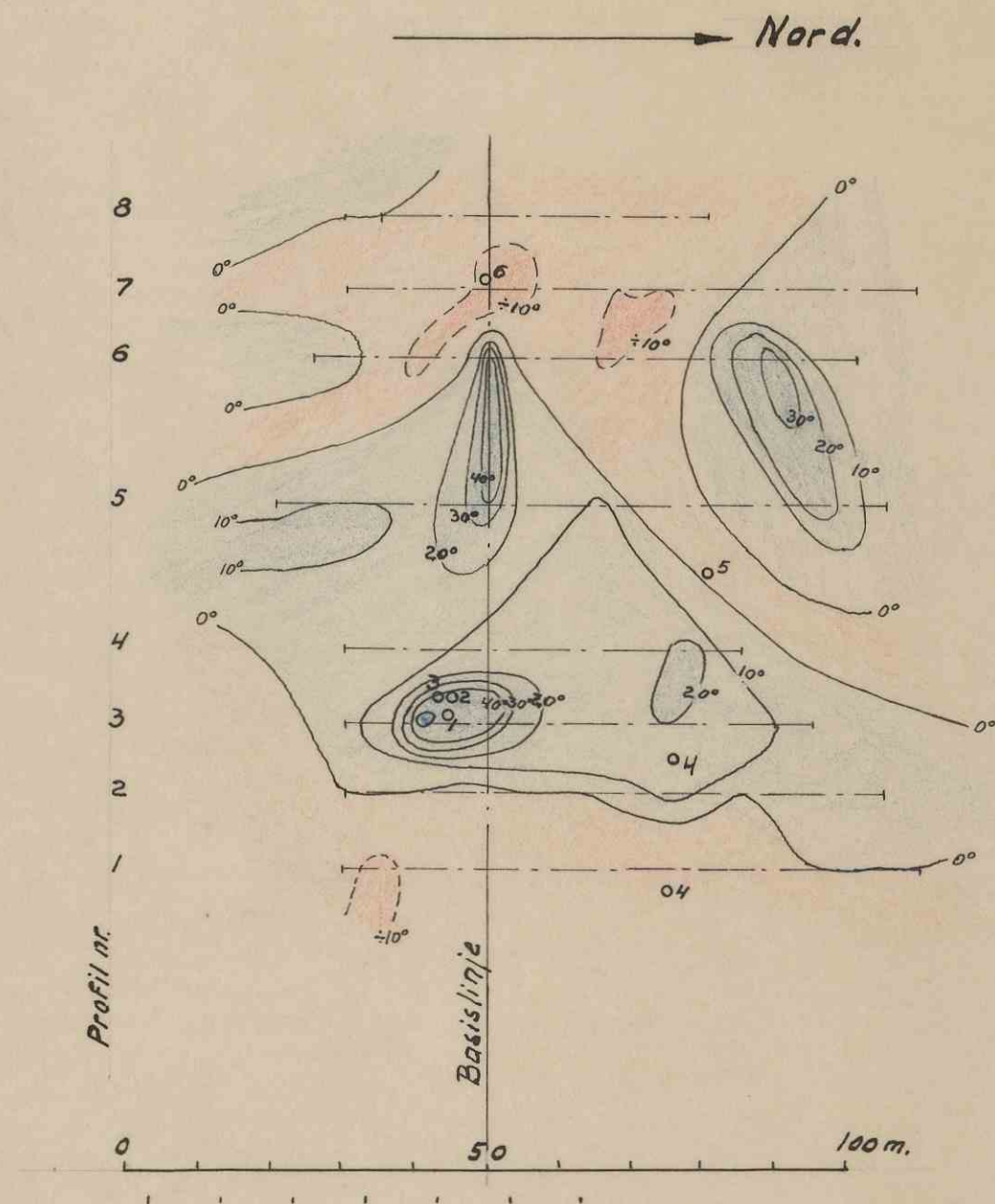
Vertikalintensitetskart. Ekvikurver for hver 10° utslag av nål.
