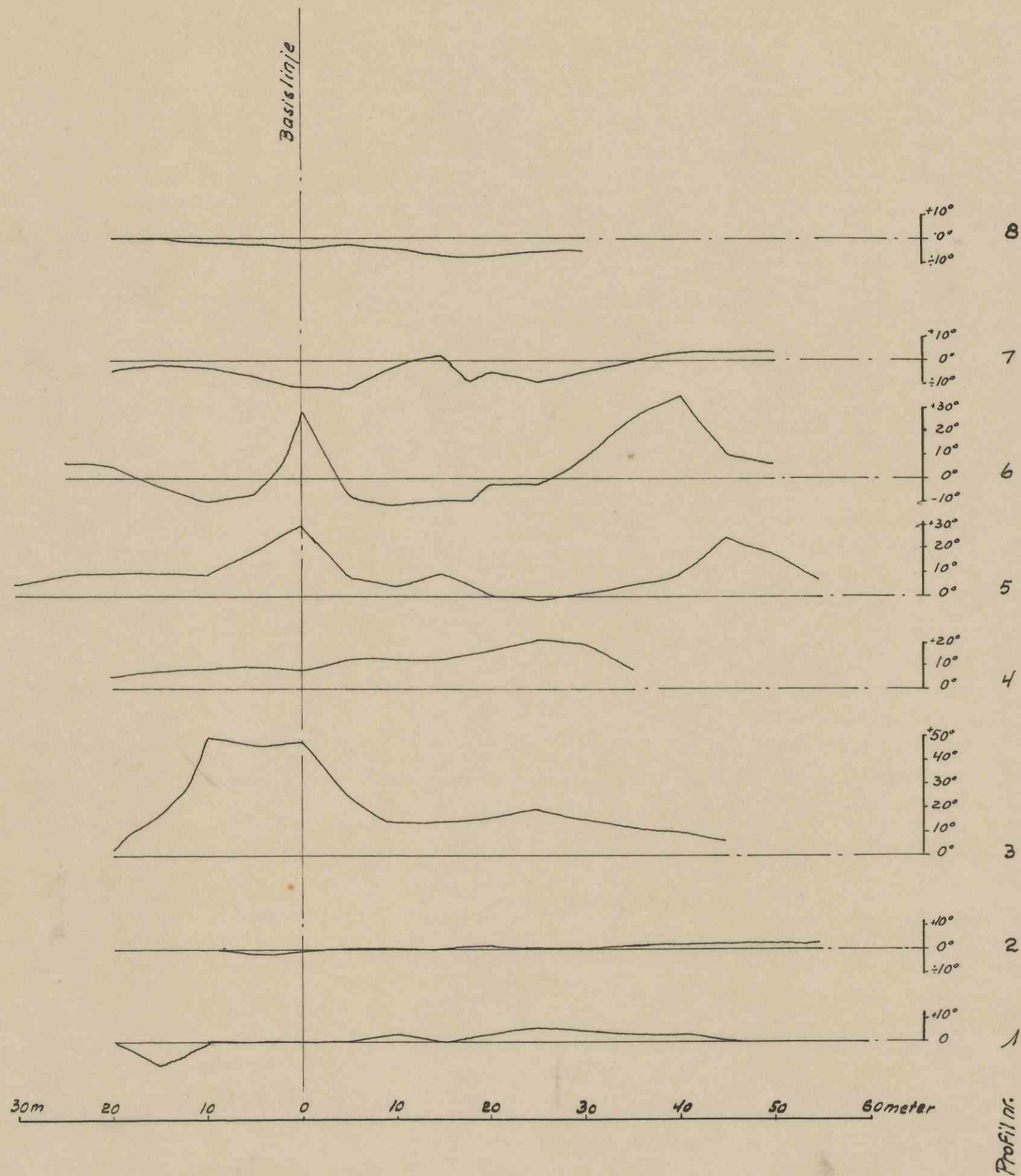
Magnetometerdrag. Nåle's utslag angitt i grader. M /500.
