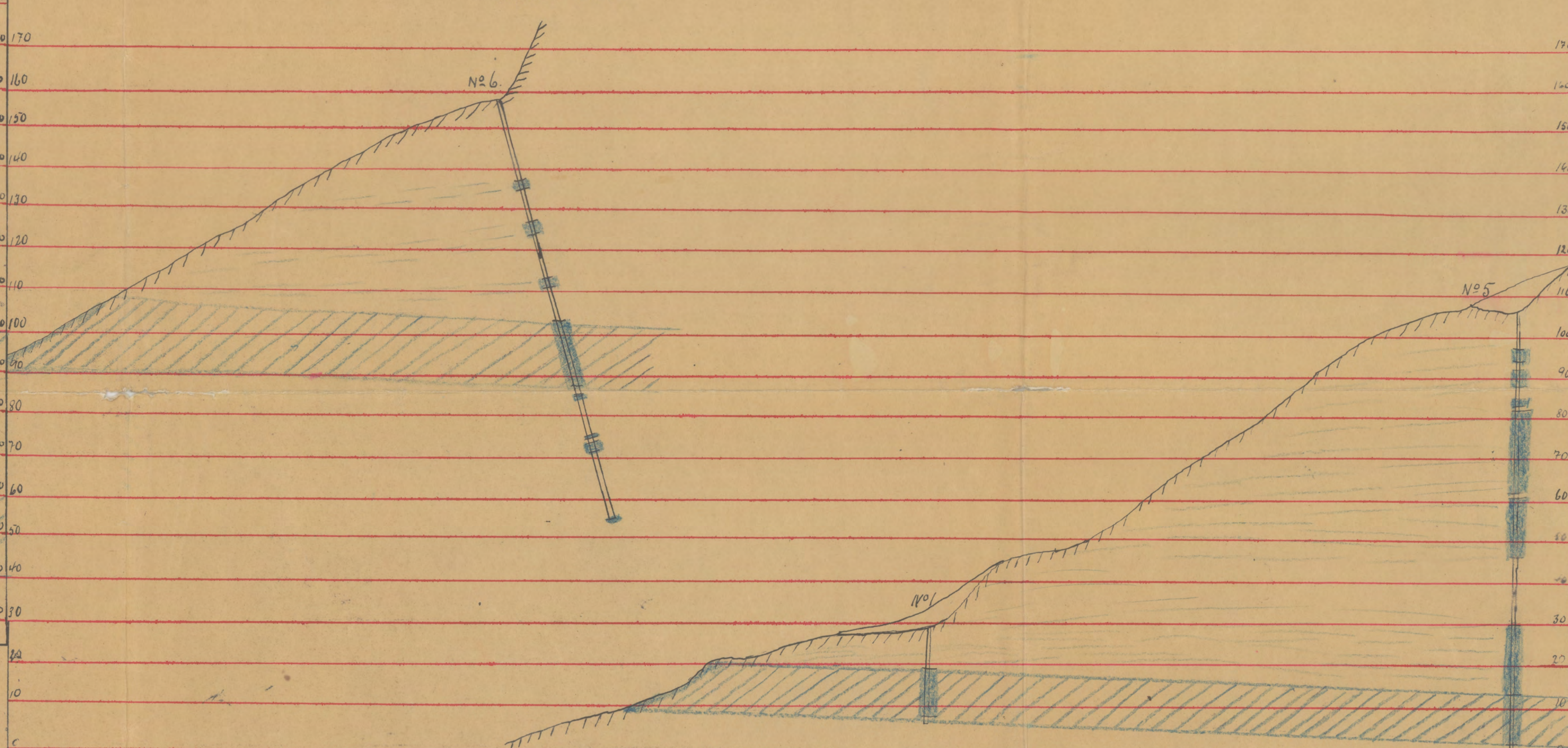
Diamantboring: Profiler av borrhuller Nr. 1, 5 & 6.
