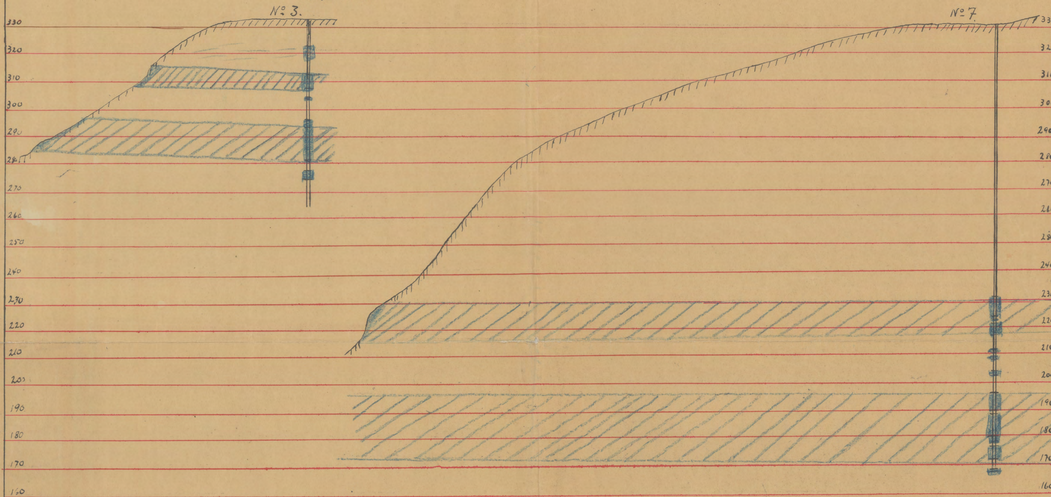
Diamantboring: Profiler av borrhuller Nr. 3 & 7.
