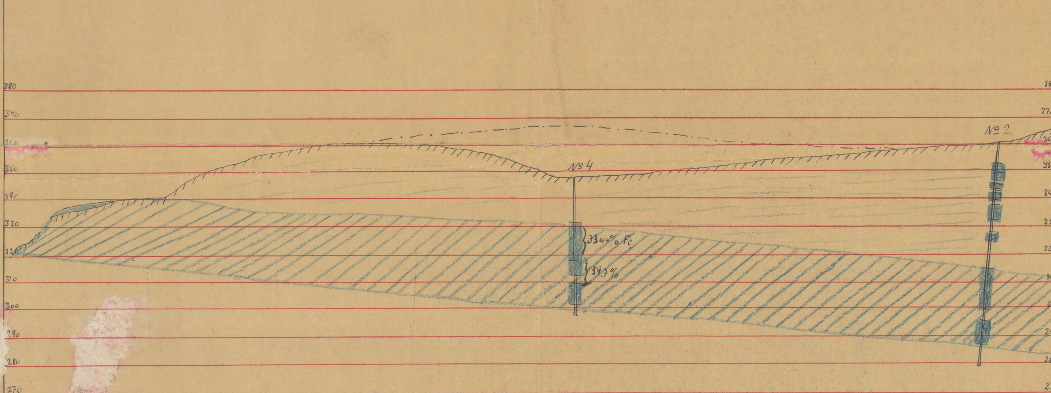
Diamantboringarna Profil av borrhålen N° 2 & 4.
