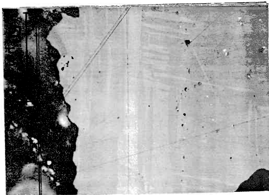
Fig. 32. Fra kvarts-feldspat mobiliseringer med molybdenglans. Kobberkis (under xN) med tvillinglameller.
