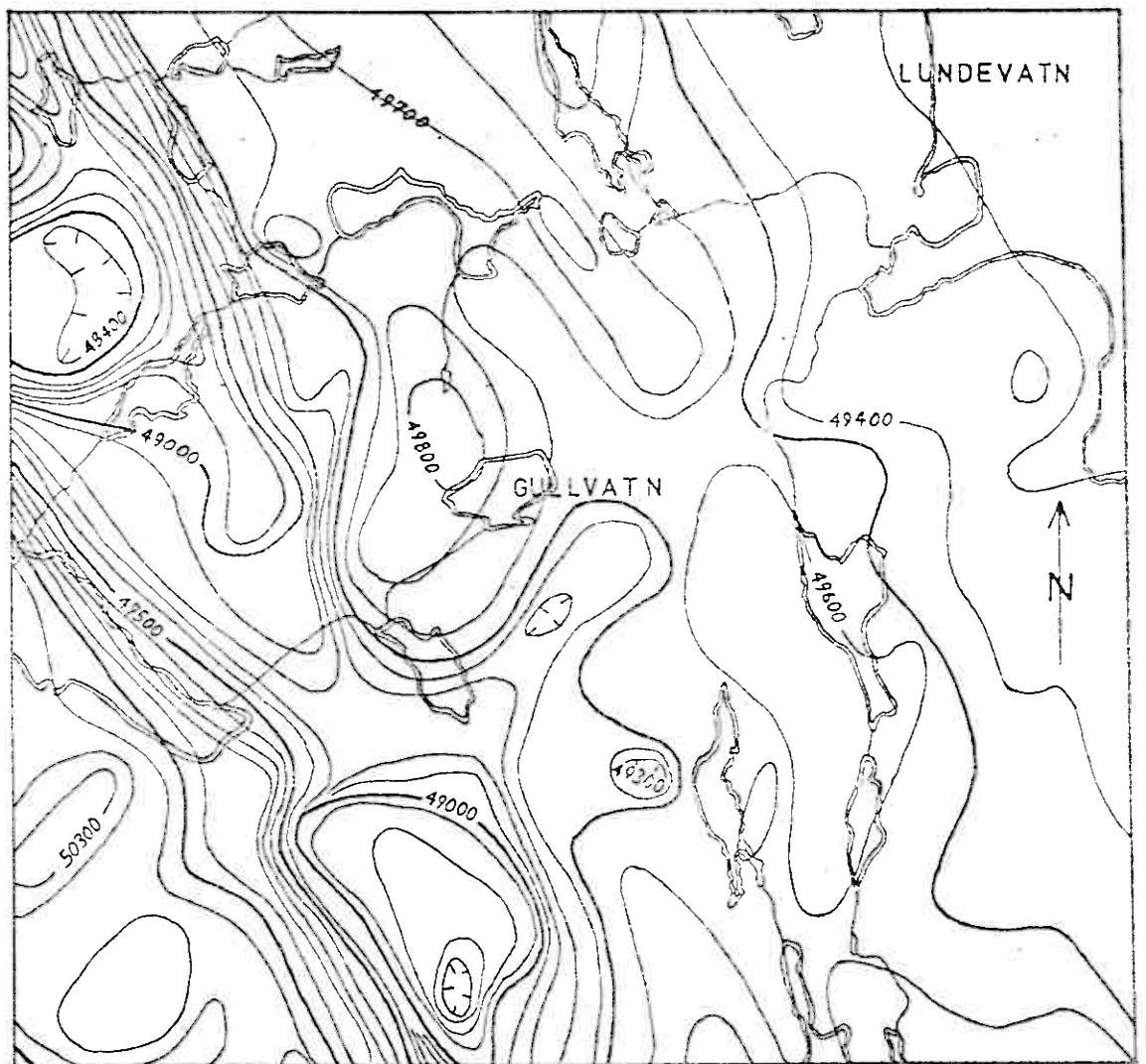
Fig. 3. Udsnit af aeromagnetisk kort 1311 IV, Sokndal i målestokken 1:50.000 (udgivet af NGU).
