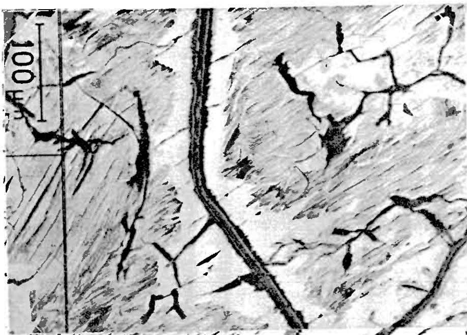
Fig. 41. Fra kvarts-feldspat mobiliseringer med molybden-glans. Magnetkis der udviser "bird-eye" tekstur.
