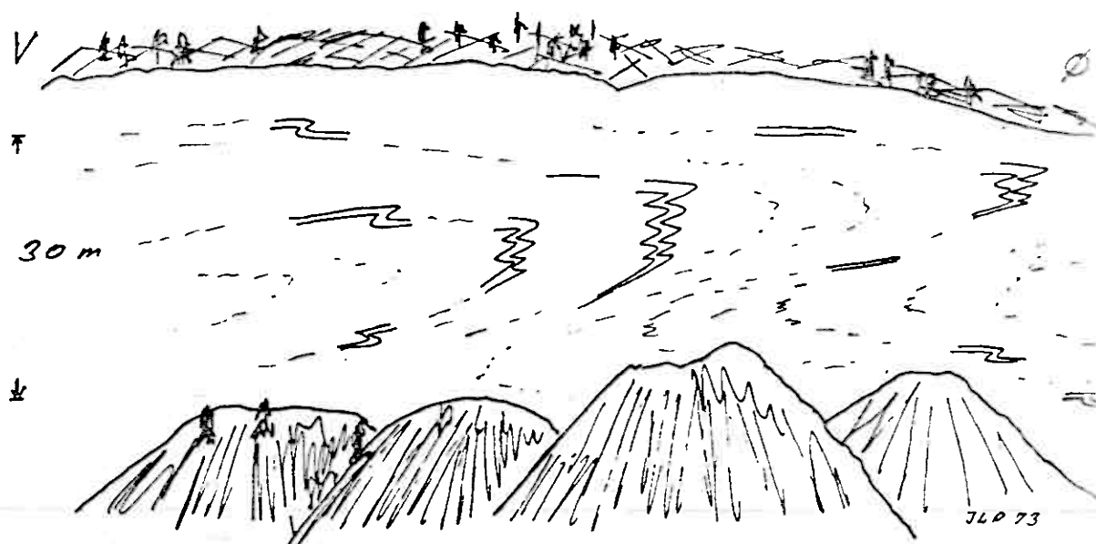
Fig. 26. Profil af stejlvæg umiddelbart nordøst for Gullbergsknuten. Fladtliggende isoklinale folder.
