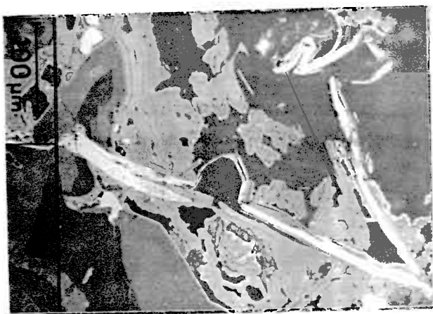
Fig. 29. Hypersten gnejs. Tråde af molybdenglans i limonit. Limoniten har replaceret pyrit.
