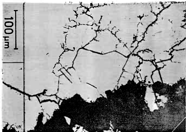
Fig. 38. Fra kvarts-feldspat mobiliseringer med molybdenglans. I et uregelmæssigt opsprækket pyritkorn findes der indslutninger af tre guldauddiskorn (lidt mørkere) xM.
