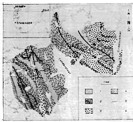
Fig. 45. Oversigtskort over Gursli-Sira områderne. Med rødt er indtegnet aksialplanssporet for de isoklinale folder. Legende: Kvarts-feldspat gnejs (1), båndet gnejs (2), sjeagnejs (3), anorthosit (4), bjergartsgrænser (5) og grænse for karterede område (6).
