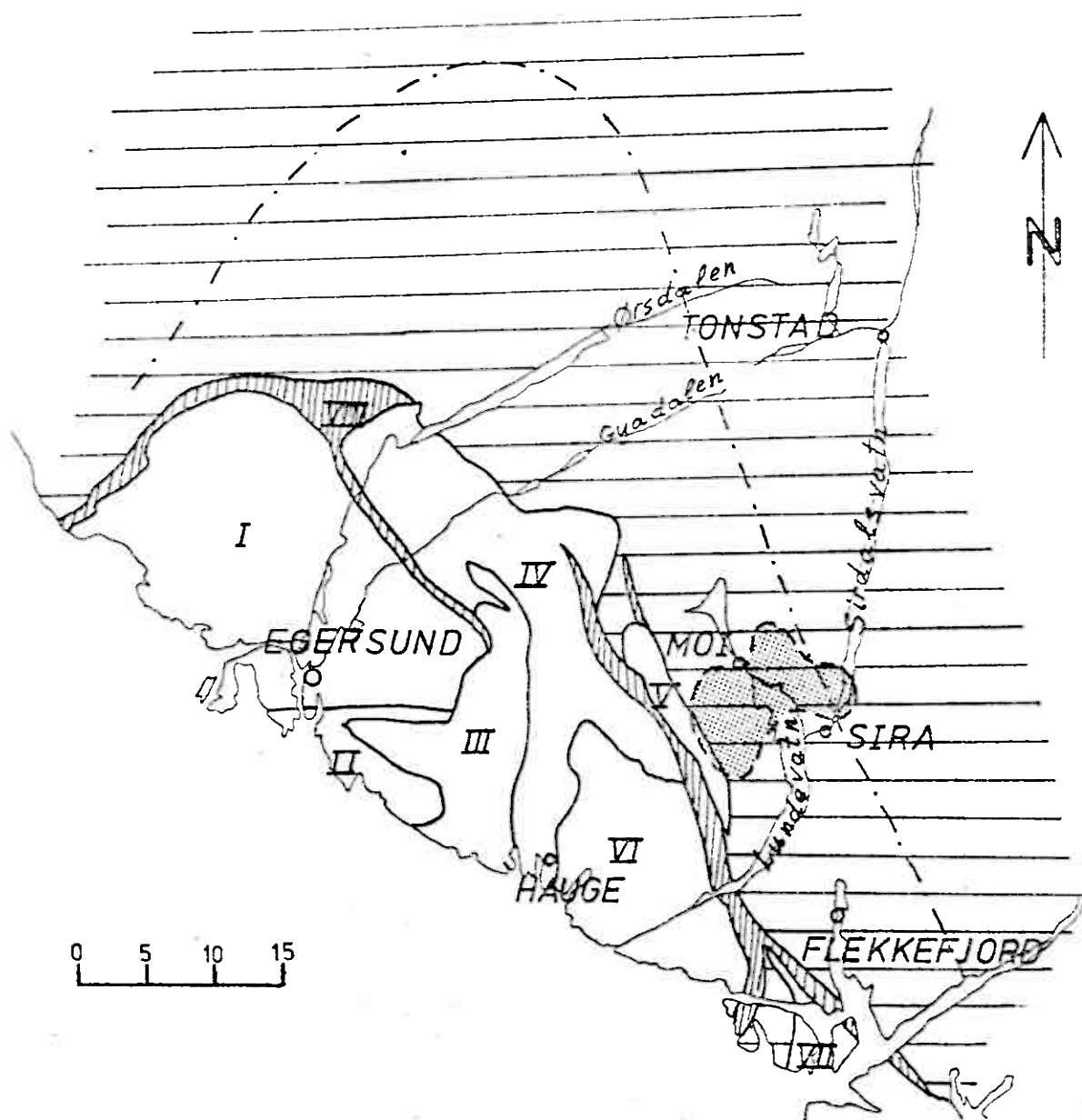
Fig. 2. Geologisk oversigtskort over SV-Norge efter BARTH (1960). Forklaring til signaturerne gives i teksten.
