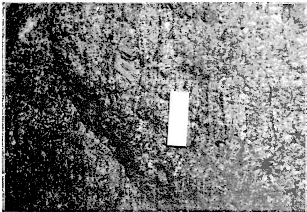
Fig. 20. Øjegnejs. Man ser, hvorledes foliationen bøjer rundt omkring feldspatmegakrysterne. Målestokken er 3 cm.
