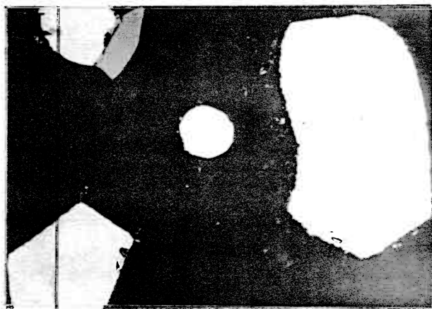
Fig. 17. Sulfidmineraler fra pyroxenit. Til højre er der et magnetkiskorn med pentlanditflammer. I øverste venstre hjørne findes der et lille korn, der består af pyrit og kobberkis.
