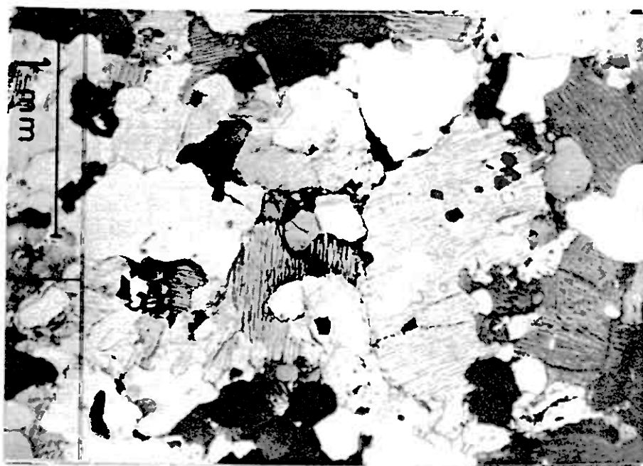
Fig. 8. Prøve fra området øst for Storestemmen. Sammen- voksninger mellem mesoperthit og kvarts.
