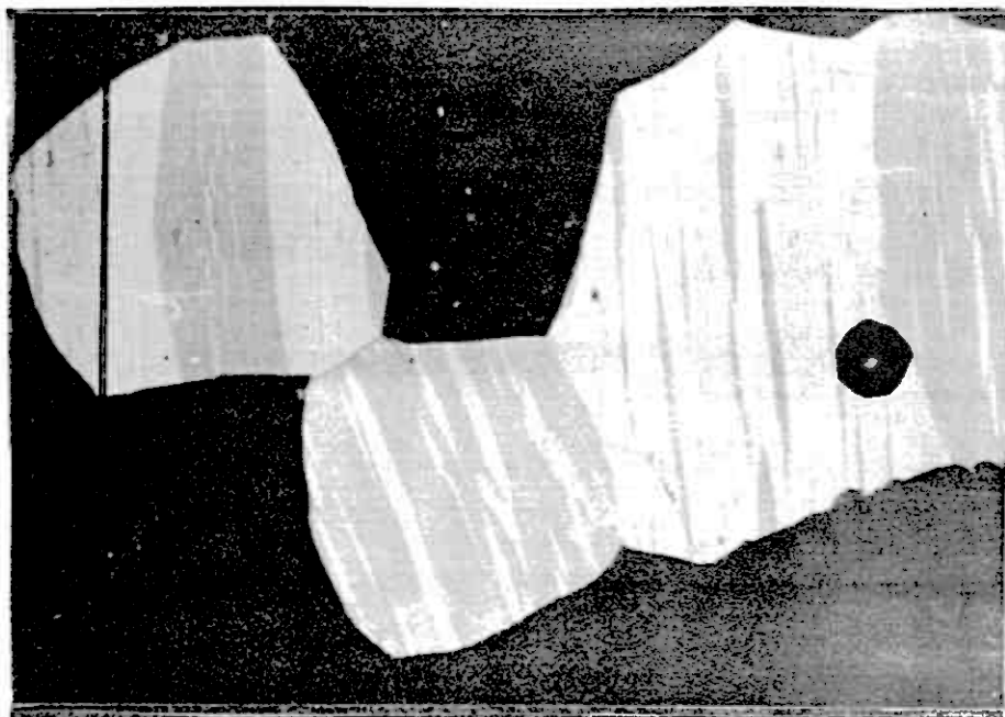
Fig. 21. Øjegneds. Afblandinger mellem hematit og ilmenit (ilmenit er det mørkeste mineral).
