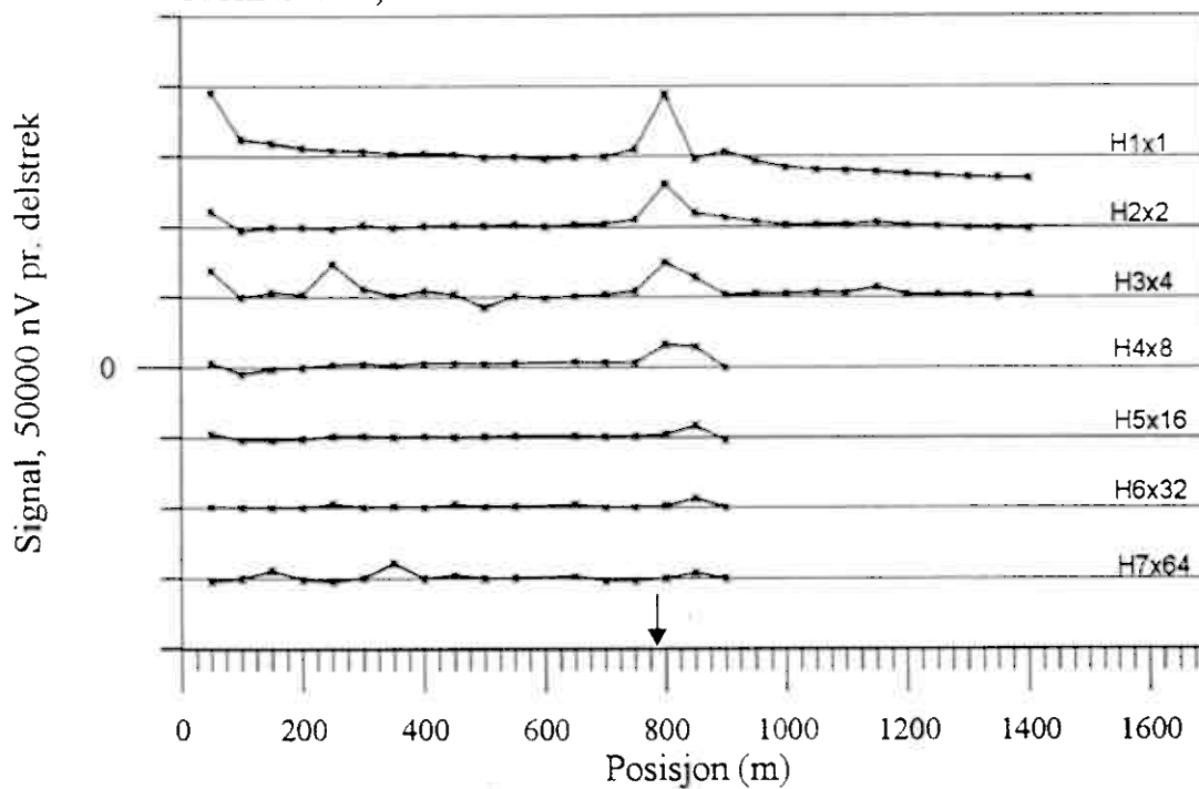
Figur 2a. Vertikal og horisontalkanaler profil 2400N
