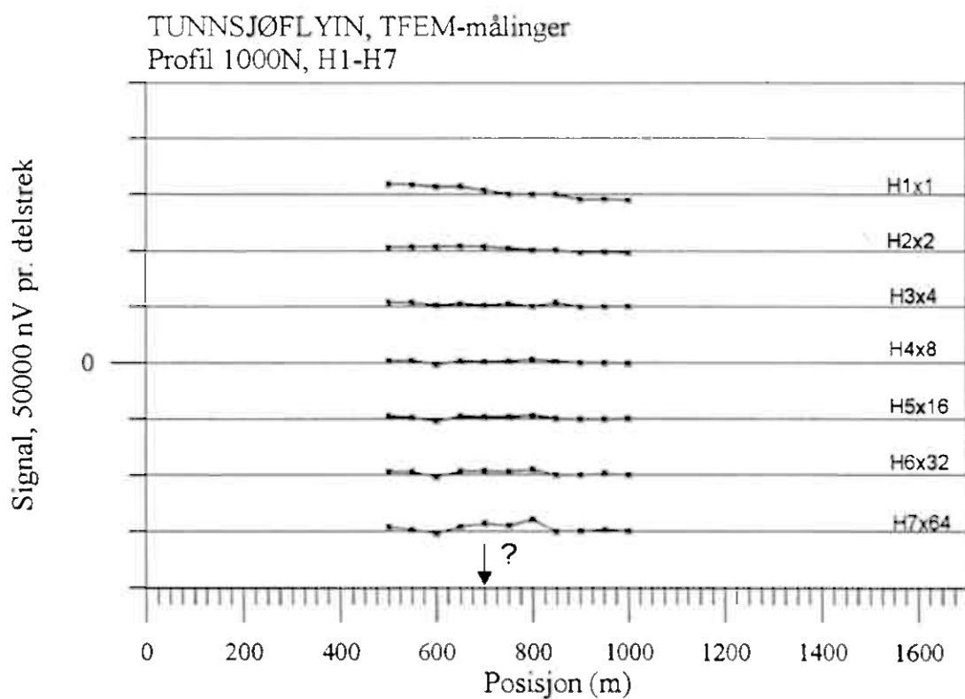
Figur 9a. Vertikal og horisontalkanaler profil 1000N
