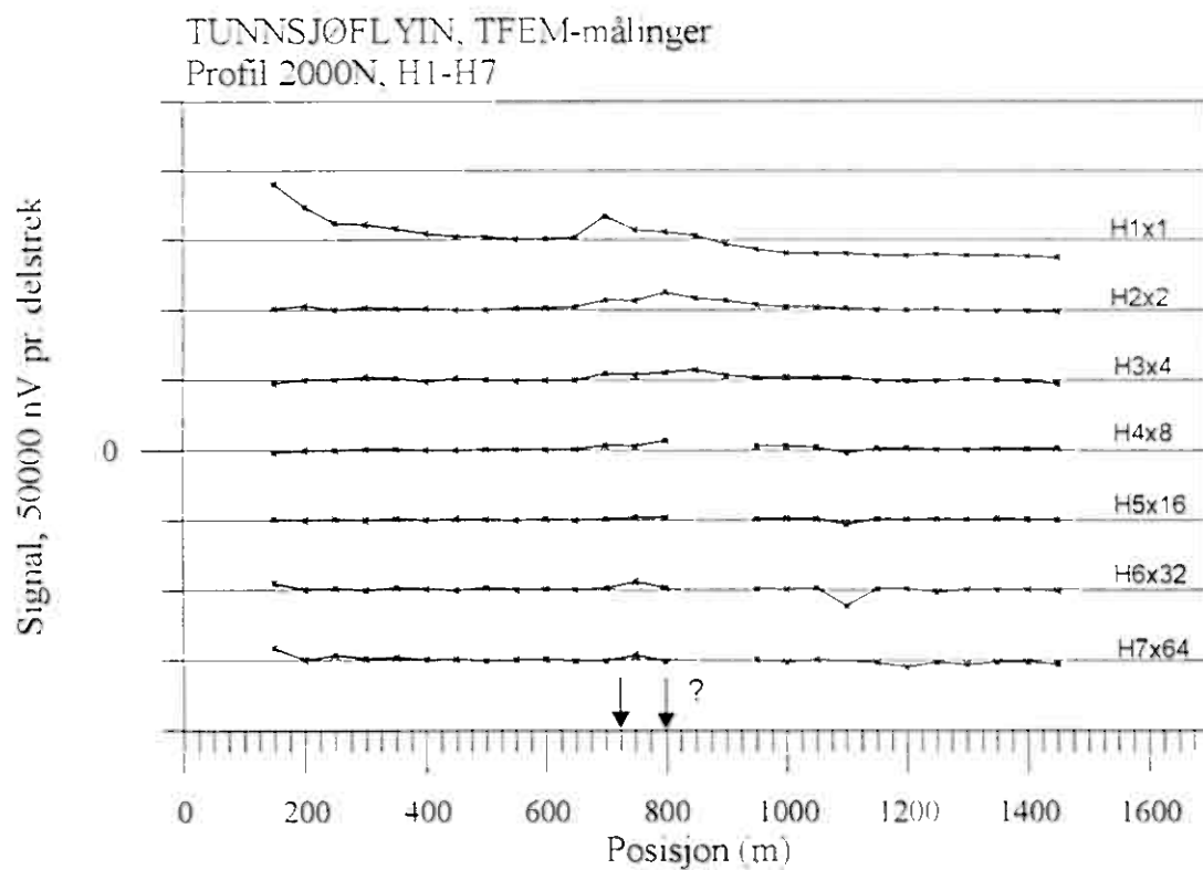
Figur 4a. Vertikal og horisontalkanaler profil 2000N
