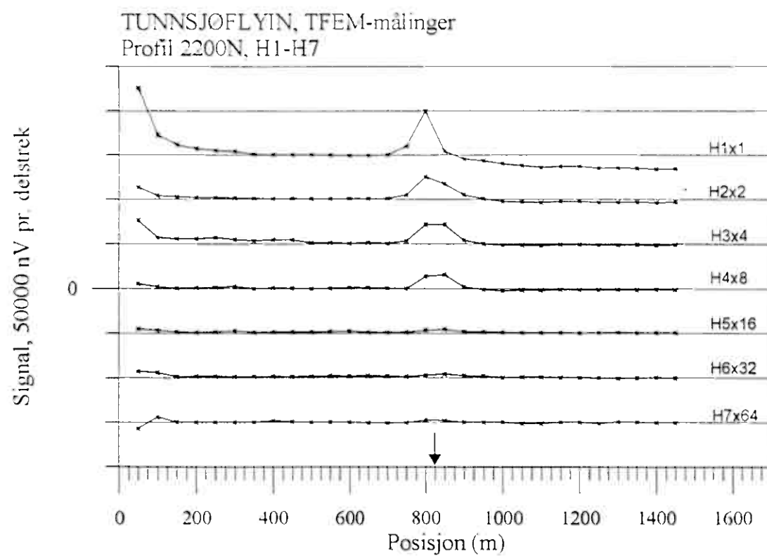
Figur 3a. Vertikal og horisontalkanaler profil 2200N
