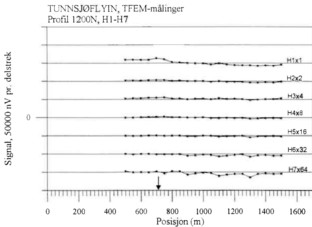
Figur 8a. Vertikal og horisontalkanaler profil 1200N
