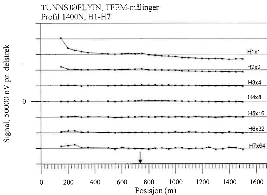
Figur 7a. Vertikal og horisontalkanaler profil 1400N
