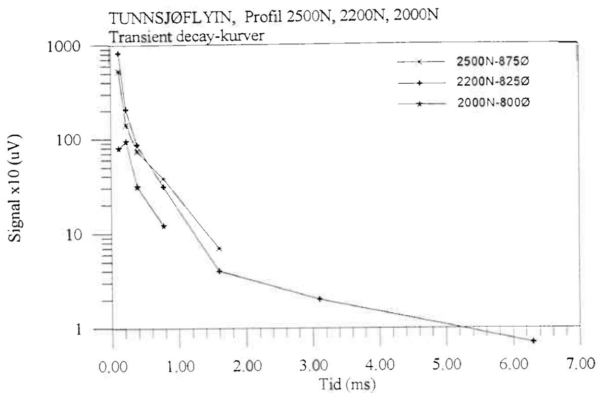
Figur 10. Transient decay-kurver for H1- H7 for leder på profil 2500N, 2200N og 2000N
