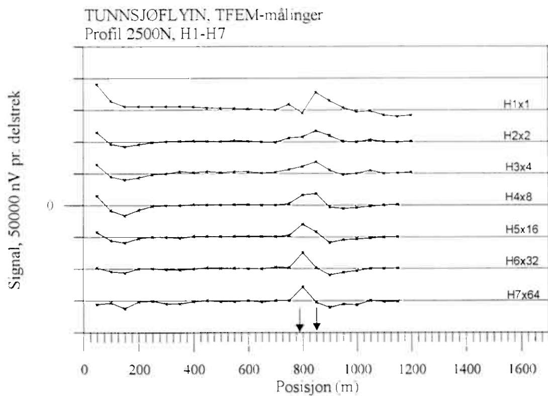
Figur 1a. Vertikal og horisontalkanaler profil 2500N
