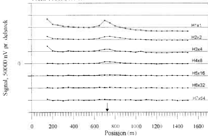
Figur 5a. Vertikal og horisontalkanaaler profil 1800N
