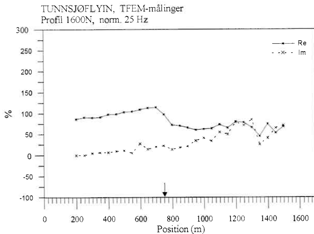
Figur 6b. Normalisert V0, Htot og 25 Hz, profil 1600N
