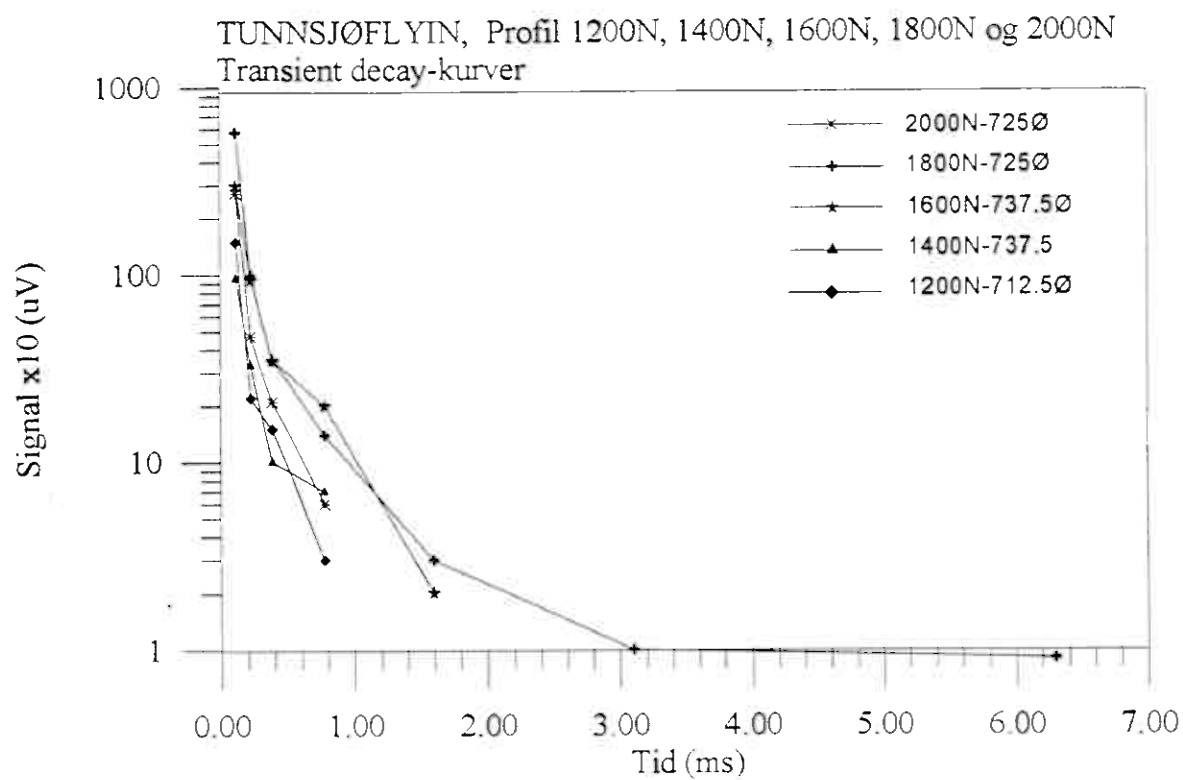
Figur 12. Transient decay-kurver for H1- H7 for leder på profil 1200N, 1400N, 1600N, 1800N og 2000N.
