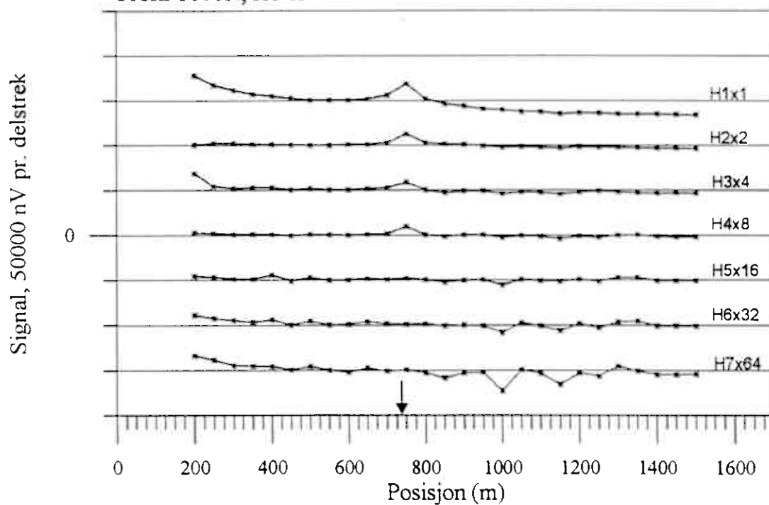
Figur 6a. Vertikal og horisontalkanaler profil 1600N
