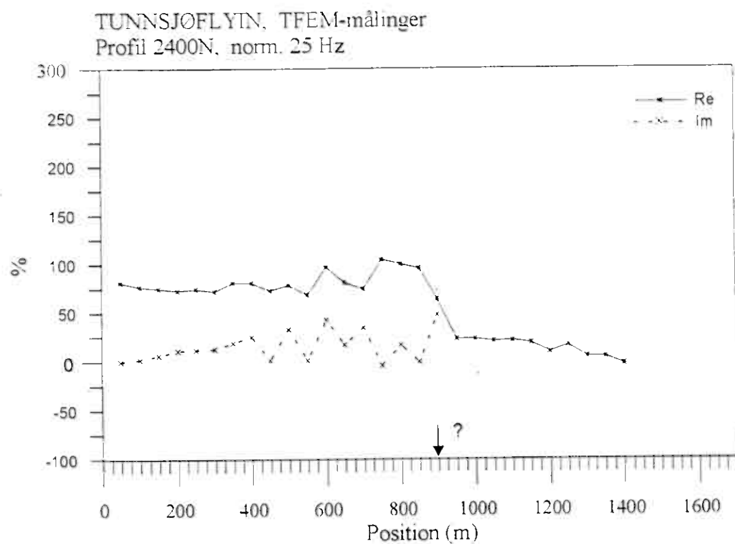
Figur 2b. Normalisert V0, Ht og 25 Hz, profil 2400N
