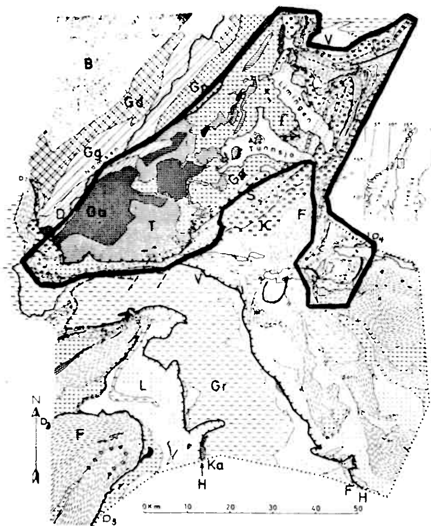
Geologisk kartskisse over Grongfeltet, Grong-kulminasjonen og Trondheimsfeltet i sørvest. Etter Chr. Oftedahl (1956).
