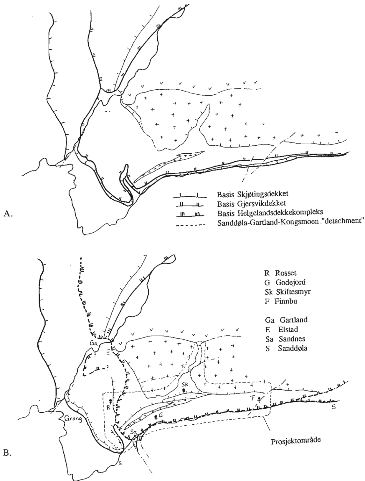
Figur 1. Tektonostratigrafien i det sørvestlige hjørnet av Grongfeltet: A. Etter dagens geologiske kart (Roberts & Reinsbakken 1991) B. Etter forfatterens undersøkelser Prosjektområdet er avmerket i B.
