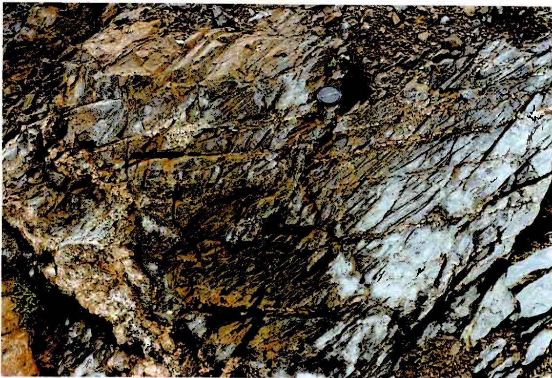
Figur 9. Karbonatomvandlet grønnstein fra den østlige del av hovedskjerpet på Sordalshøgda.
