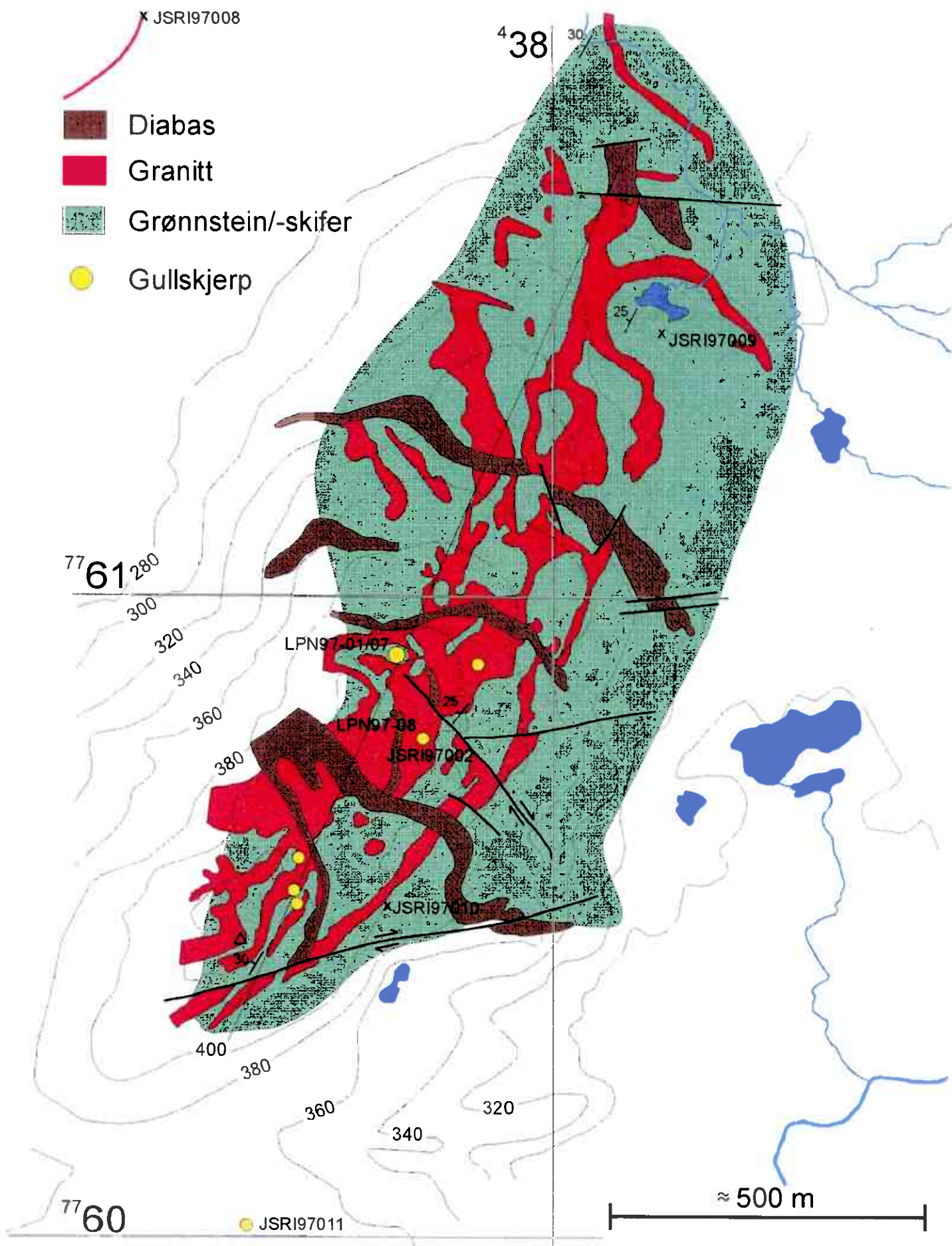
Figur 4. Berggrunnskart over Sordalshøgda platået, forenklet fra Lieungh (1985, Bilag 9). Hovedskjerp er det nordvestre gullskjerp og lengst i sør er rustsonen med Au-Zn-Ag mineralisering påvist av Folldal Verk A/S avmerket (Kap. 3.4). Provelokaliteter og foliasjon fra undersøkelsene i 1997 er i tillegg vist. Målestokk og UTM-lokalisering er omtrentlige.
