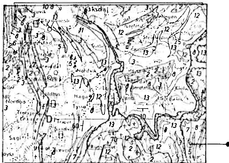
Figur 2 Utsnitt av 1:250.000 berggrunnsgeologisk kart Bergen
