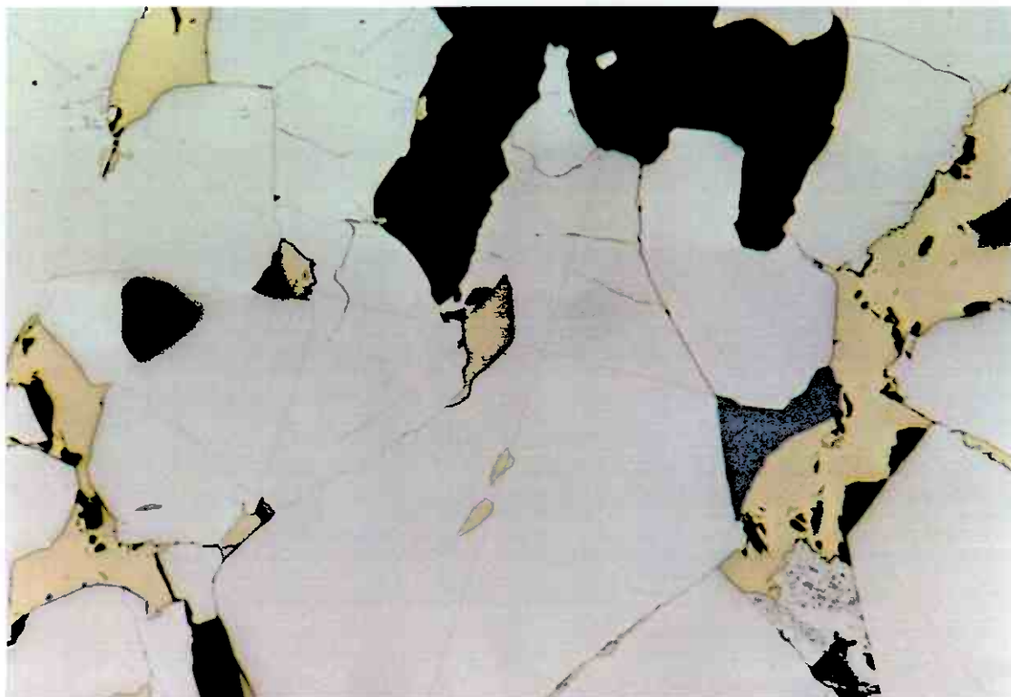
Figur 21. SR 08. Skiftesmyr. Lys gul svovelkis, gul kobberkis og grå zinkblende. Bildets bredde ca. 2 mm.
