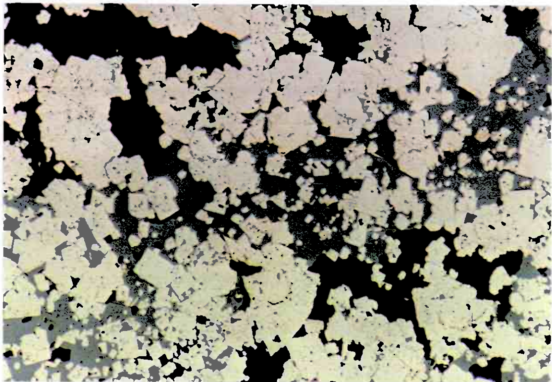
Figur 13. JA 17. Joma. Pålys. Lys gul svovelkis og grå zinkblende. Bildets bredde ca. 2 mm.
