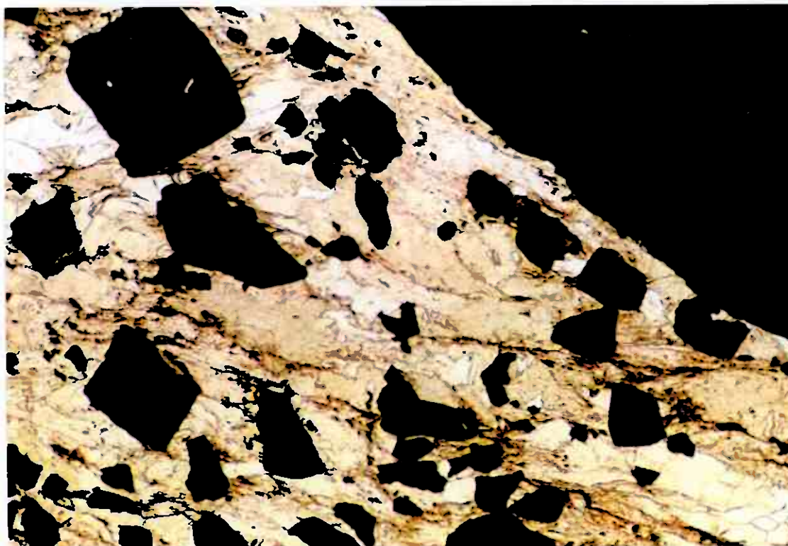
Figur 9. SR 17. Skiftesmyr. Gjennomfallende lys. Man ser her hvordan den hvite kvartsen og lysegrønne kloritten er tektonisert. De svarte eriskornene (svovelkis) er brukket i stykker. Bildets bredde er ca. 4 mm.
