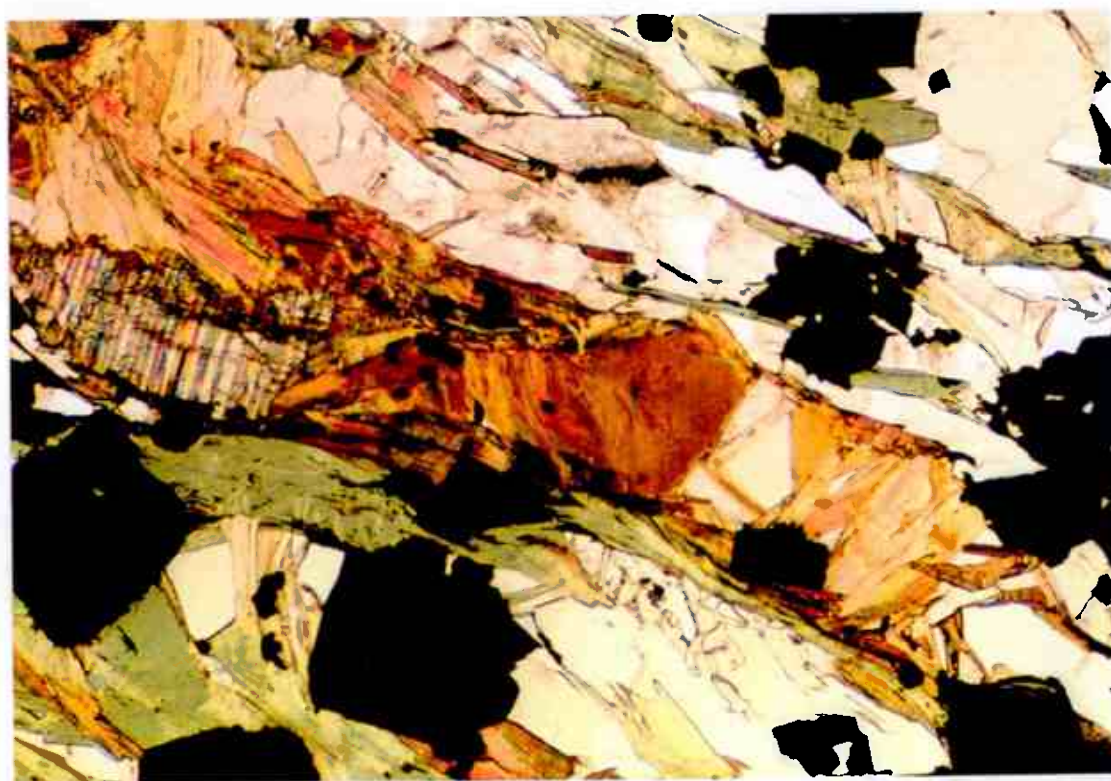
Figur 17. TT 08. Tverrfjellet. Gjennomfallende lys. Brun biotitt, grønn kloritt og til venstre i bildet et karbonatkorn med parallelle tvillingstriper. Bergarten har vært tektonisert. Kvartsen er helt lys mens ertsen er svart. Bildets bredde er ca. 2 mm.
