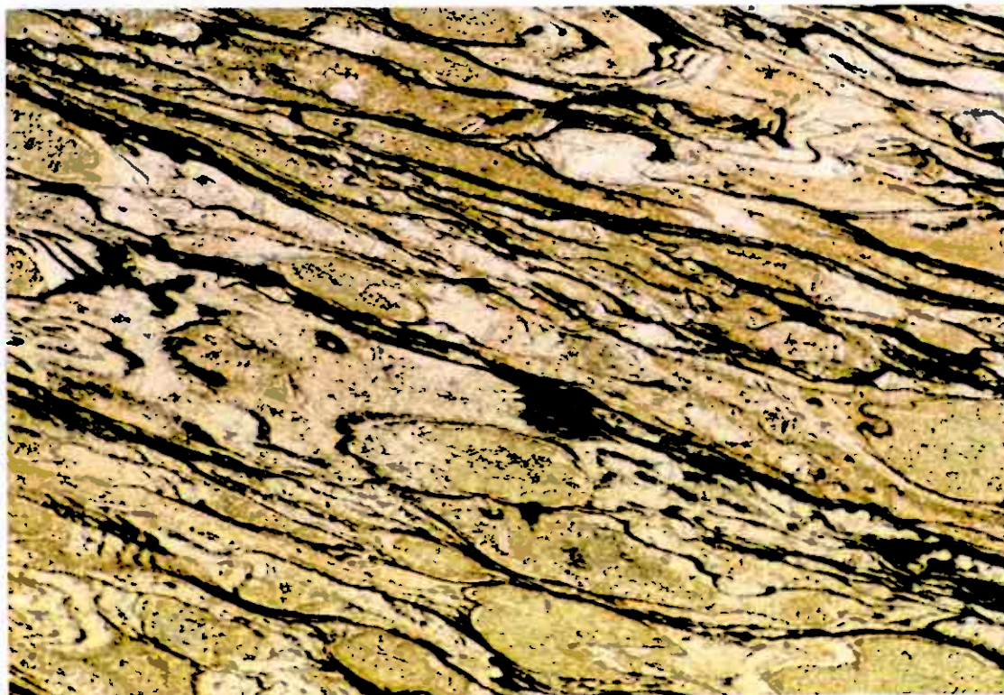
Figur 6. LN 09. Løkken. Sterkt mylonittisert og foldet bergart. På grunn av den ekstremt lave kornstørrelsen er det vanskelig å skille de enkelte mineralene, men de lysegrønne partiene består vesentlig av kloritt. Bildets bredde er ca. 4 mm.
