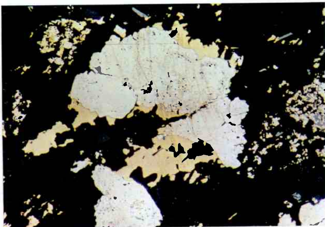
Figur 16. LN 19. Løkken. Pålys. Lys gul svovelkis og gul kobberkis. Bildets bredde ca. 2 mm.
