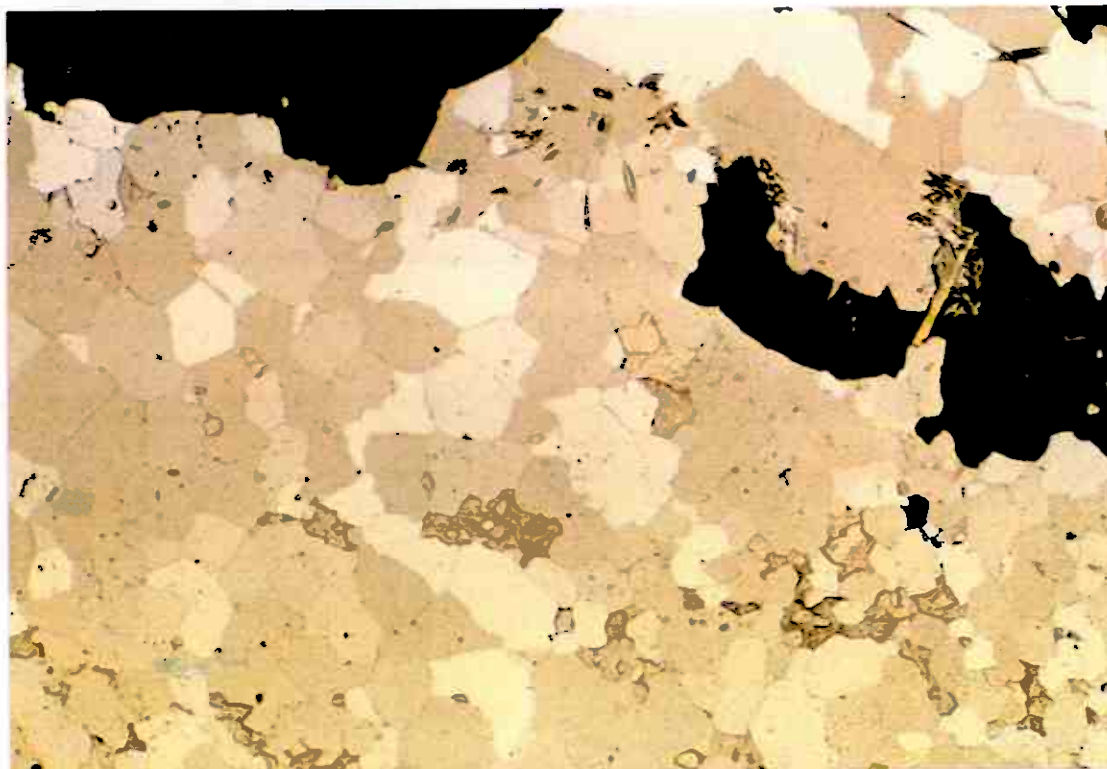
Figur 4. JA 10a. Joma. Lyse eller beige korn av kvarts/sur plagioklas, ofte har disse rette korgrenser, mens de brune spredte karbonatkornene har uregelmessige korgrenser. Svart erts. Bildets bredde er ca. 4 mm.
