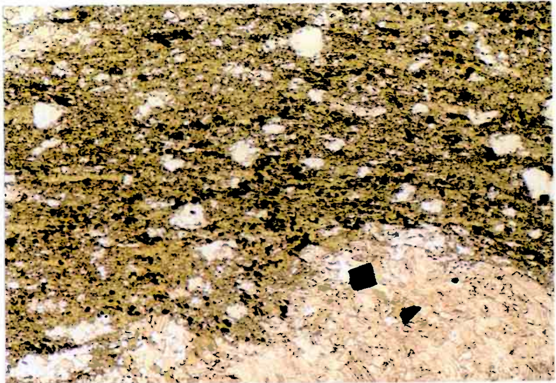
Figur 1. SS 20. Skorovass. Matrix består for det meste av grønn kloritt, lysere kvarts og svart erts. Større lyse korn er kvarts. I nedre del av bildet sees del av en karbonatlinse, i denne sees også to større svarte ertskorn. Bildets bredde er ca. 4 mm.
