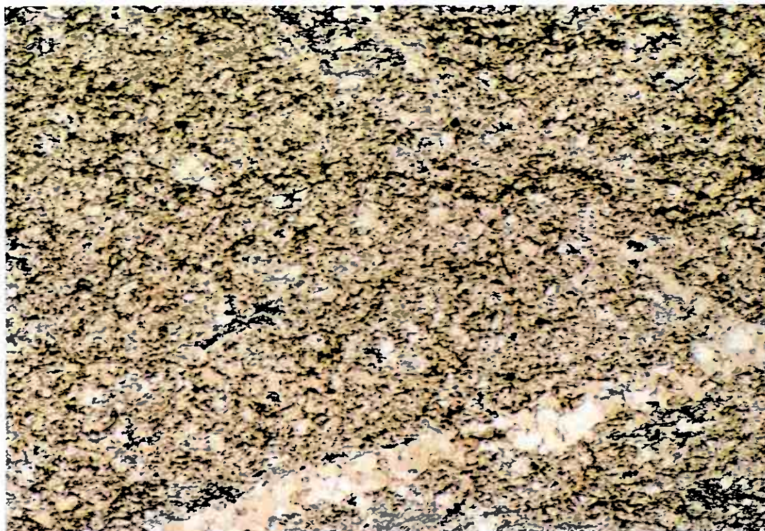
Figur 3. GK 06. Gjersvik. Blanding av kvarts og kloritt. De lyseste kornene er kvarts, mens de mørkere er enten kloritt, kvarts eller karbonat. I den nedre del av bildet sees et bånd med hvit kvarts og beige karbonat. Bildets bredde er ca. 4 mm.
