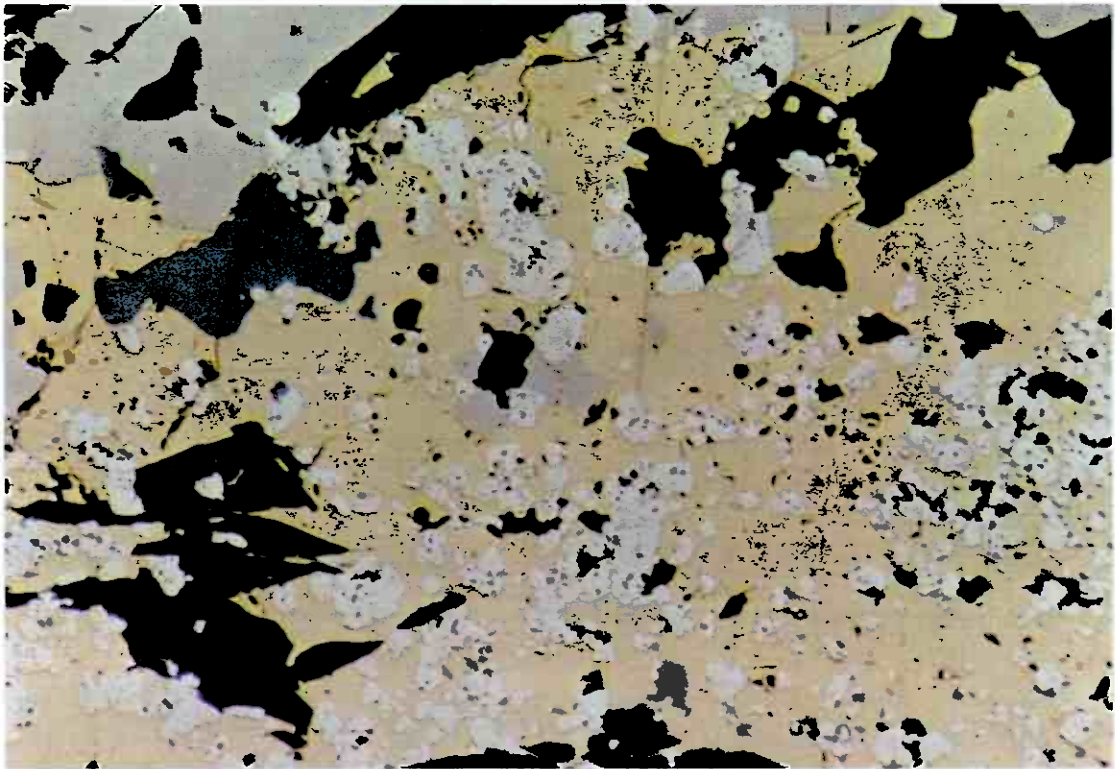
Figur 12. JA 08. Joma. Pålys. Gul kobberkis, lys gul svovelkis, grå zinkblende og beige magnetkis. Bildets bredde ca. 2 mm.
