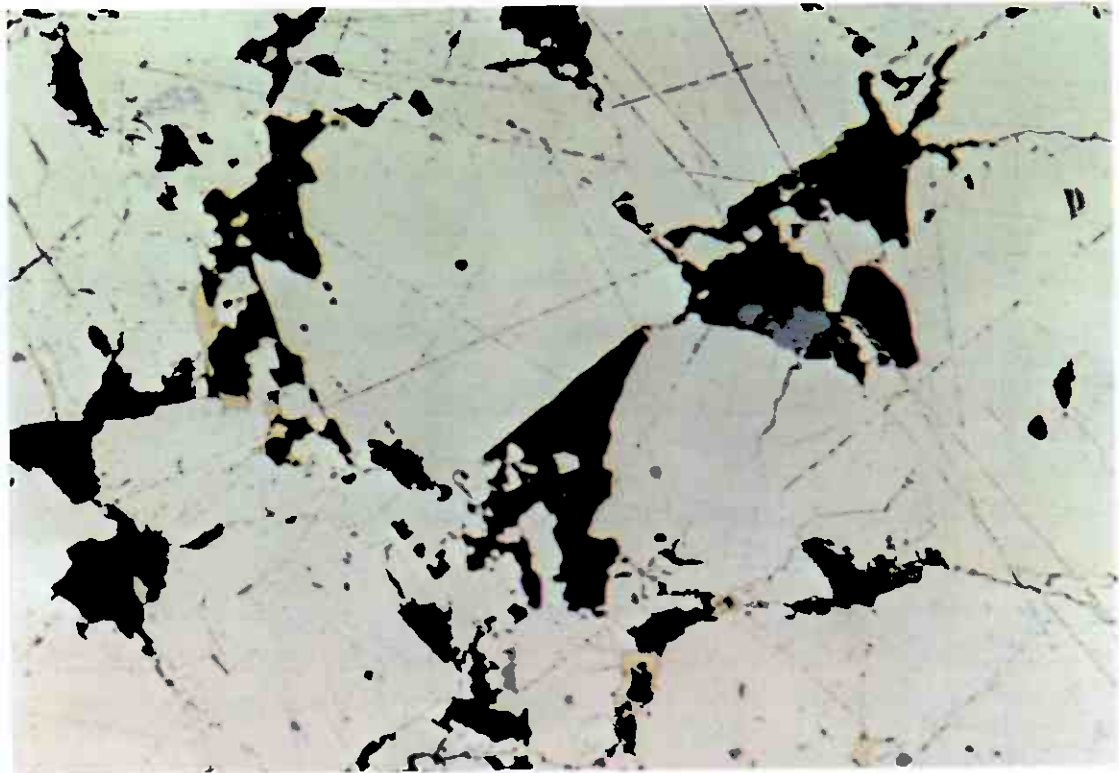
Figur 25. TT 04. Tverrfjellet. Lys gul svovelkis, gul kobberkis og grå zinkblende. Bildets bredde ca. 2 mm.
