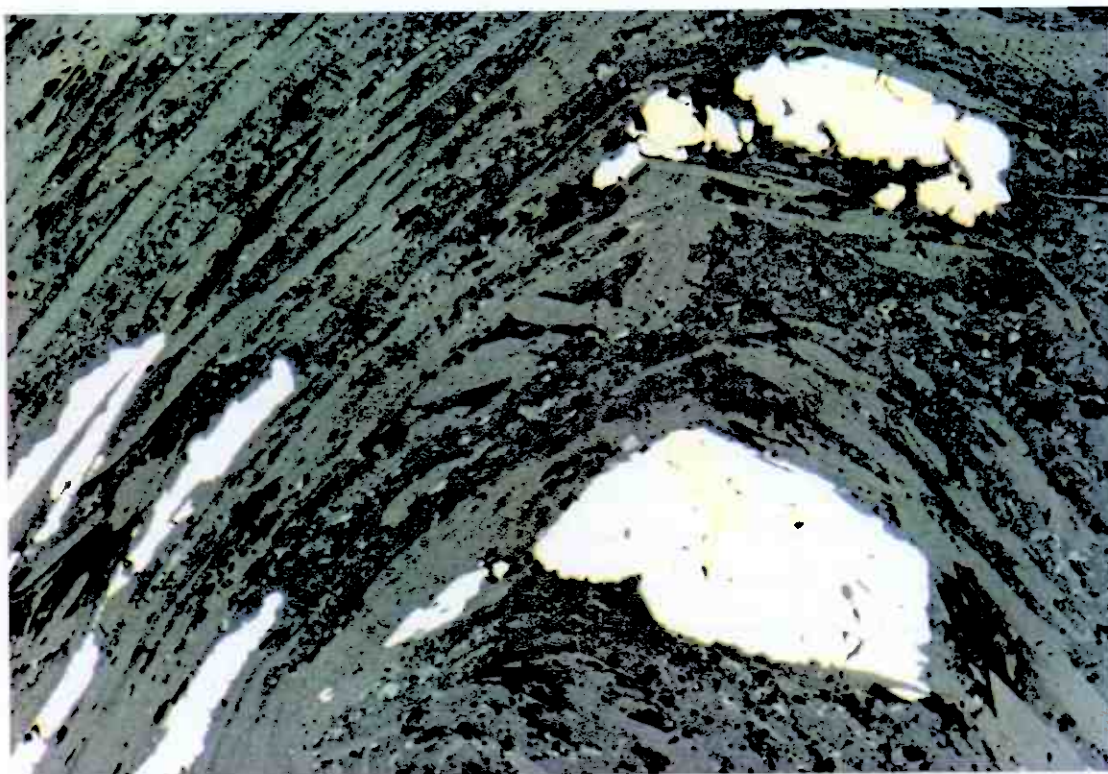
Figur 14. JA 18. Joma. Pålys. Beige magnetkis og gul kobberkis i en foldet bergart. Man ser også hvordan kisen er tynnet ut på siden av folden. Bildets bredde ca. 2 mm.
