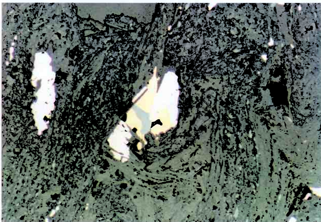
Figur 15. JA 18. Joma. Pålys. Som på fig. 14, her også beige magnetkis og gul kobberkis, men her også sammen med grå zinkblende. Bildets bredde ca. 2 mm.
