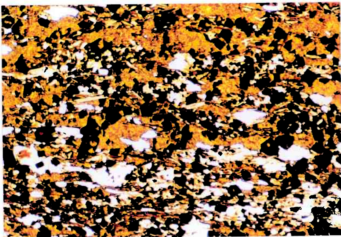
Figur 10. GK 04. Gjersvik. Gjennomfallende lys. Brun, noe grumset zinkblende mens de svarte svovelkiskornene er ugjennomsiktige. De lyse mineralene er for det meste karbonat. Bildets bredde ca. 4mm.
