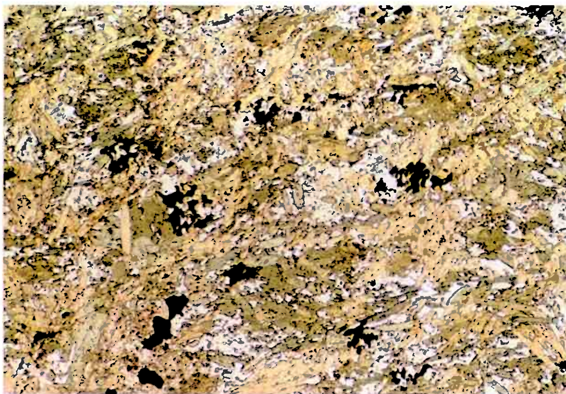
Figur 7. TT 19. Tverrfjellet. De lyseste kornene er kvarts. De lyse brungrønne og grønne kornene er vesentlig hornblende med litt karbonat som her er vanskelig å skille ut. Svart er pyrit. Bildets bredde er ca. 4 mm.
