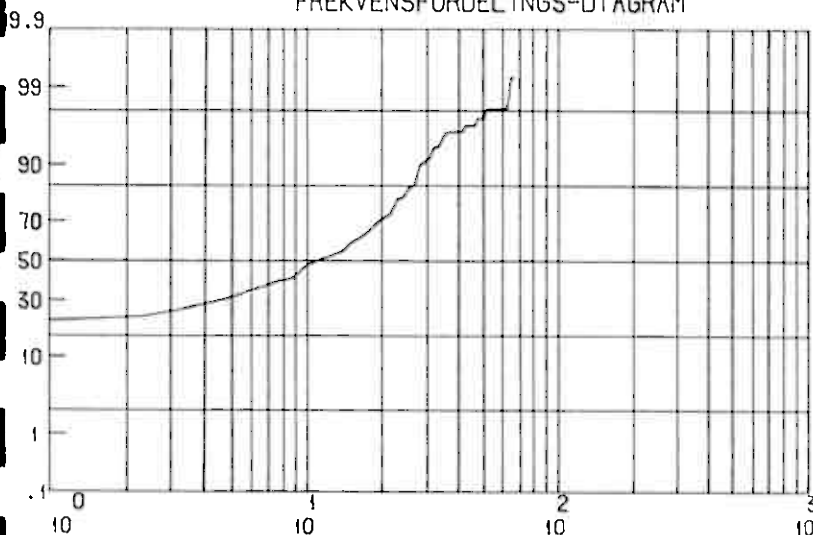
FREKVENSFORDELINGS-DIAGRAM
