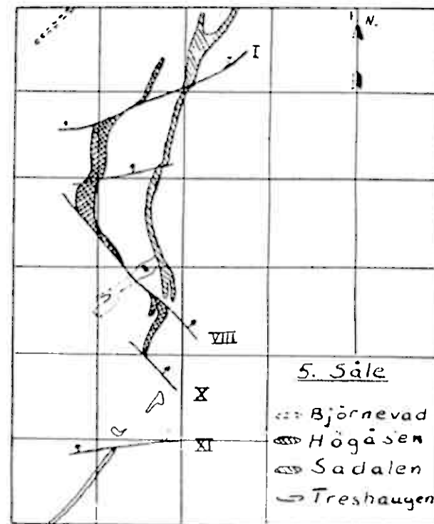
Horisontalsnitt av kisingangane på 5. sale.
