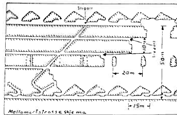
Vertikalsnitt av drift i kisingang.
