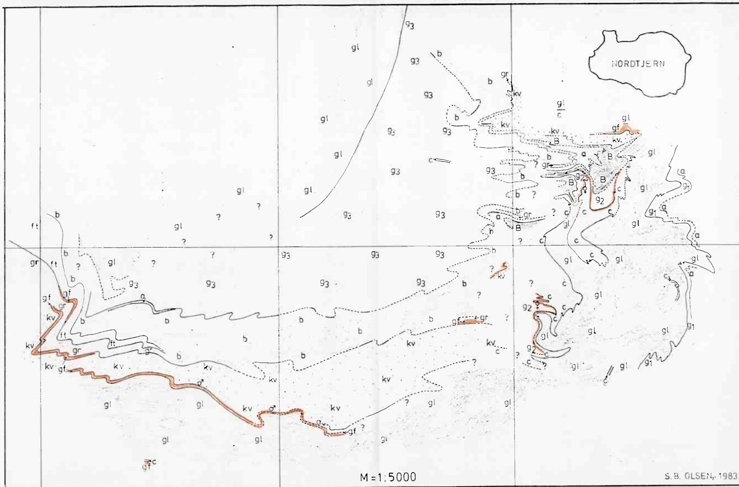
NORDTJERNBEKKEN GEOLOGISK OVERSIGTSKORT BILAG 1
