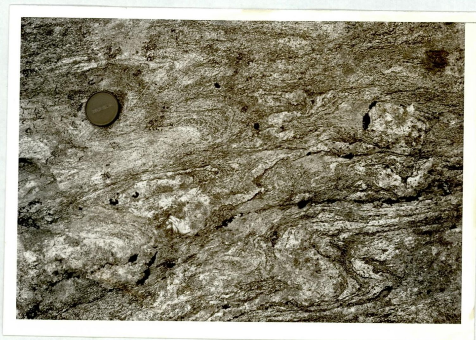
Foto 3: Foldet granat-biotit skifer med \text{MoS}_2 i pegmatitisk materiale og i foldelukninger. Faulevatsfjellet, H = 450 m.
