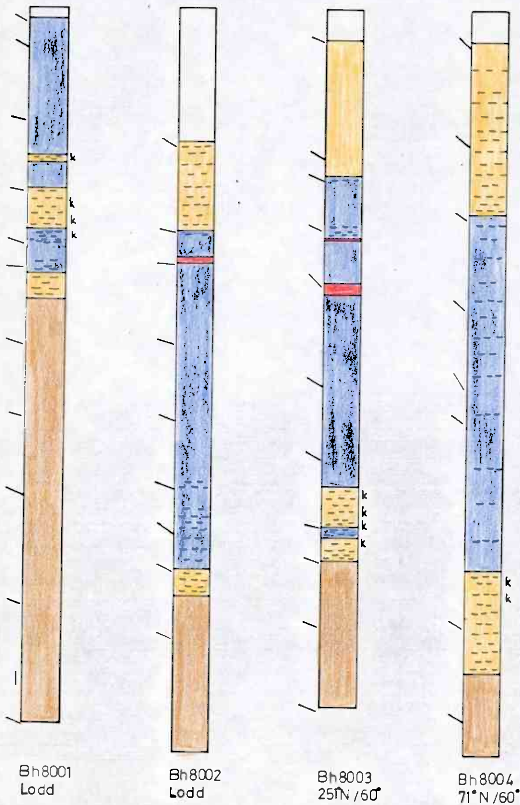
Fig. 1 a. Stratigrafi i borhull på Stödi. Tegnforklaring se fig. 1 d.
