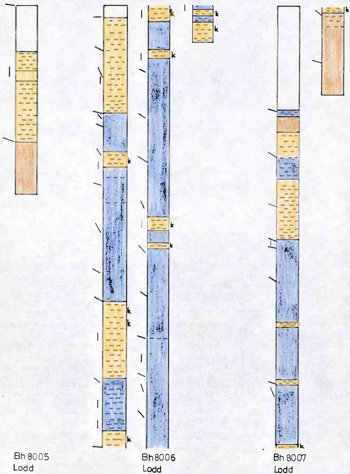
Fig. 1 b. Stratigrafi i borhull på Stødi. Tegnforklaring se fig. 1 d.
