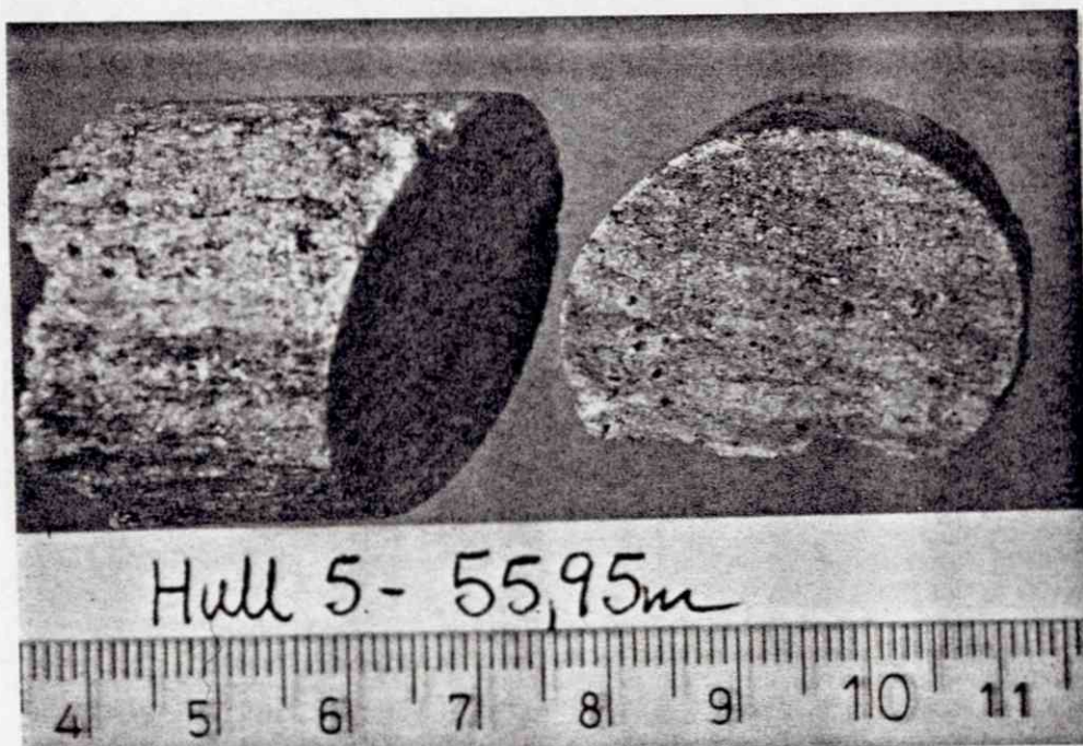
Fig. 12. Kjerneprøve hull 5 - 55,95 m. Omtrentlig mineralfordeling i tilhørende slip: ~ 30 % karbonat, 50-60 % talk, 10-15 % (?) kloritt og ~ 5 % sekundær magnetitt pluss kromitt. I slippet sees intim sammenvoksning av talk og kloritt.
