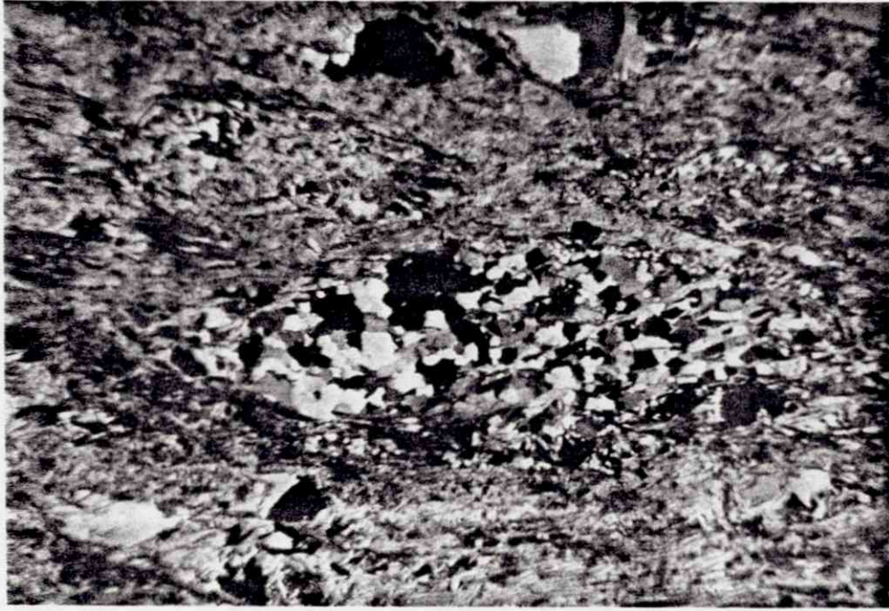
Fig. 39. Mikrofoto av slip 430 fra Råsdalsfjell.
