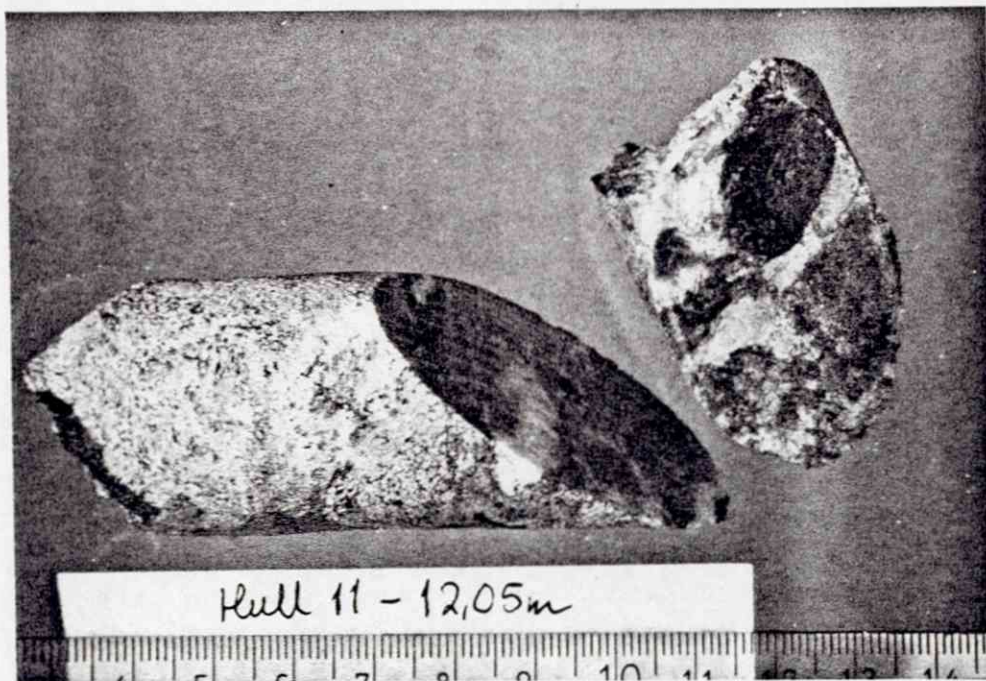
Fig. 24. Kjerneprøve hull 11 - 12,05 m. Omtrentlig mineralfordeling i tilhørende slip: ~70 % karbonat, et finkornet aggregat av ~15 % talk og ~5 % serpentinrester. Videre <5 % (?) kloritt og ~5 % sekundær magnetitt pluss kromitt. Prøven viser noe sterkere omvandling enn prøve 11 - 9,50 m. En relativ stor kromittanrikning fins i slippet. Mikrosondeanalyser nr. 8, 9, 12, 13 og 14 i Bilag 3, side 2 og 3.
