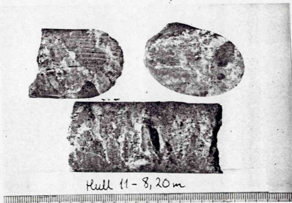
Fig. 20. Kjerneprøve hull 11 - 8,20 m. Omtrentlig mineralfordeling i tilhørende slip: ~50 % karbonat, ~25 % talk, ~20 % (?) serpentinerester, ~5 % (?) kloritt og 2-4 % sekundær magnetitt pluss kromitt. I slipet sees serpentin under omvandling til talk.
