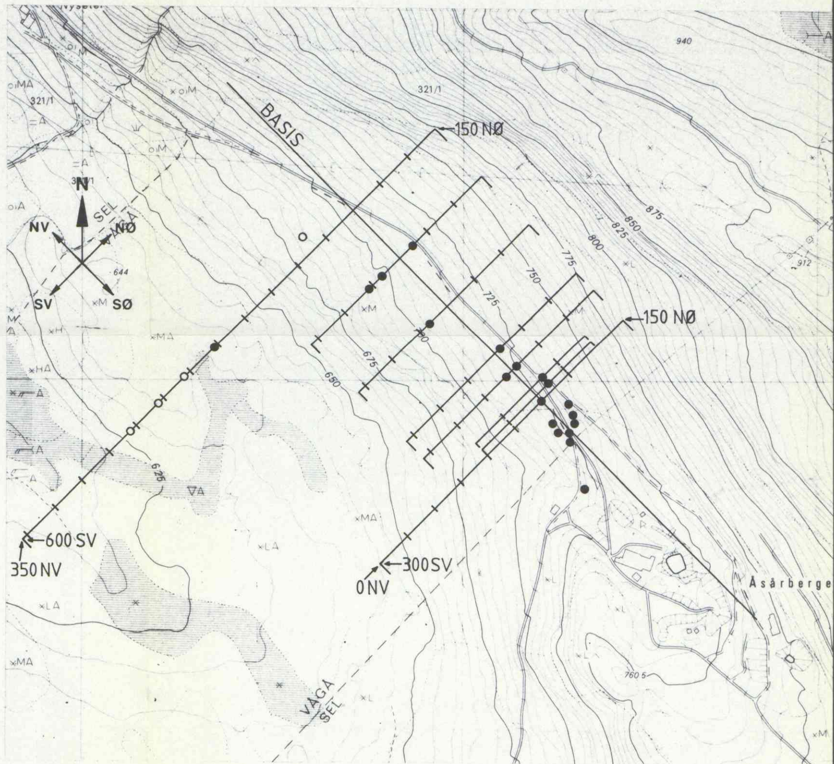
UTSNITT AV ØKONOMISK KART BW 089-5-2 RÅSDALEN MED INNTEGNING AV NØ-SV-PROFILENE I BLOKKDIAGRAMMET
