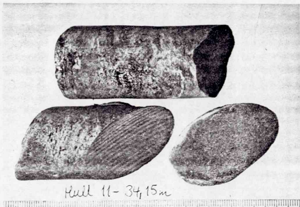
Fig. 31. Kjerneprøve hull 11 - 34,15 m.
