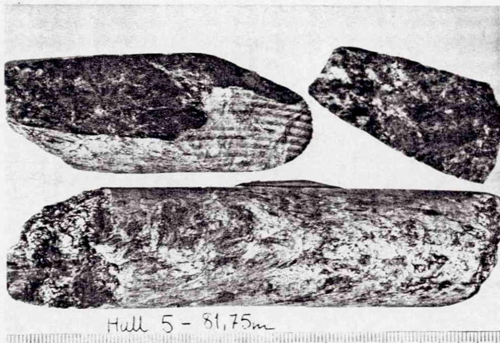
Fig. 15. Kjerneprøve hull 5 - 81,75 m. Omtrentlig mineralfordeling i tilhørende slip: ~ 40 % kloritt, ~ 40 % aktinolit, ~ 20 % talk samt aksessoriske mengder apatitt (?). Prøven er tatt fra et overgangsparti mellom kleber og klorittskifer og er derfor karakterisert ved opptreden av mye aktinolit.
