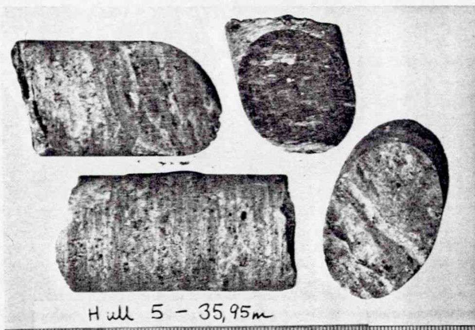
Fig. 4. Kjerneprøve hull 5 - 35,95 m. Omtrentlig mineralfordeling i tilhørende slip: ~ 20 % serpentinerester, 50-60 % talk, <10 % kloritt, ~ 20 % karbonat og 3-4 % kromitt pluss sekundær magnetitt. I slipet sees serpentin under omvandling til talk og kromittkorn med en lys brun (kromrik) kjerne og mørk (jernrik) randsone.
