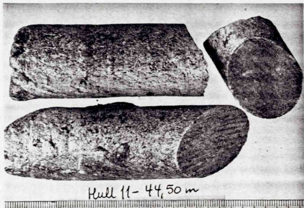
Fig. 34. Kjerneprøve hull 11 - 44,50 m.
