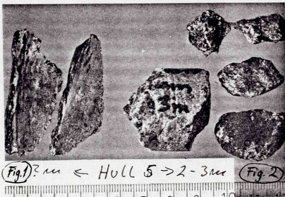
Fig. 1. Kjerneprøve hull 5 - dyp?
