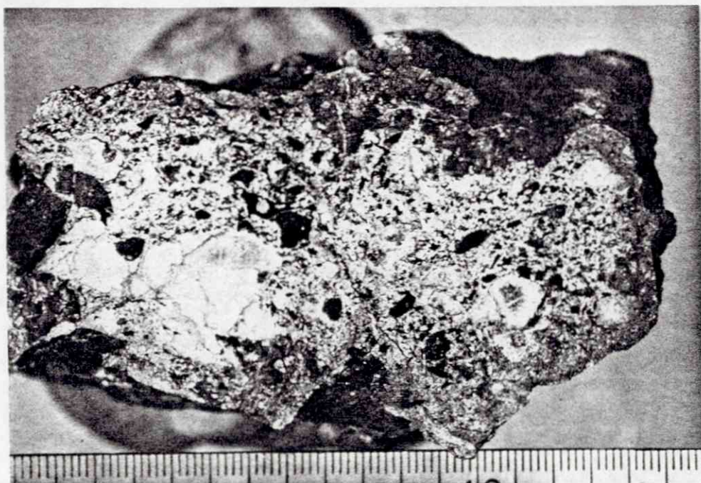
Fig. 44. Prøve nr. 170a.
