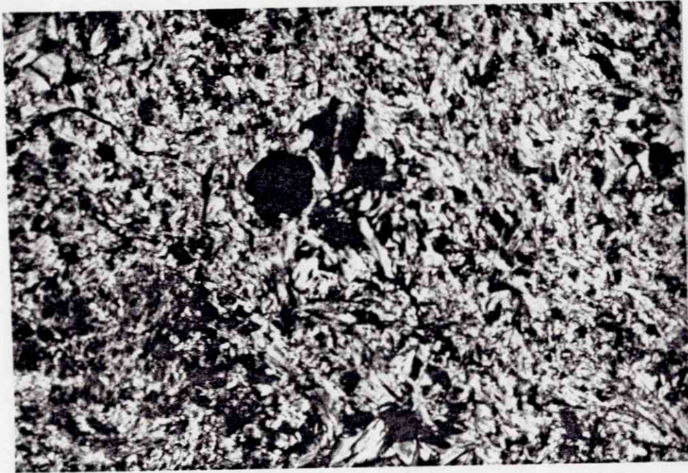
Fig. 23. Mikrofoto av slip 11 - 9,50 m. 40 x forstørrelse, kryssede nicols. En liten serpentinrest (blålig, midt på bildet) i en talk-karbonat-dominert kleber.
