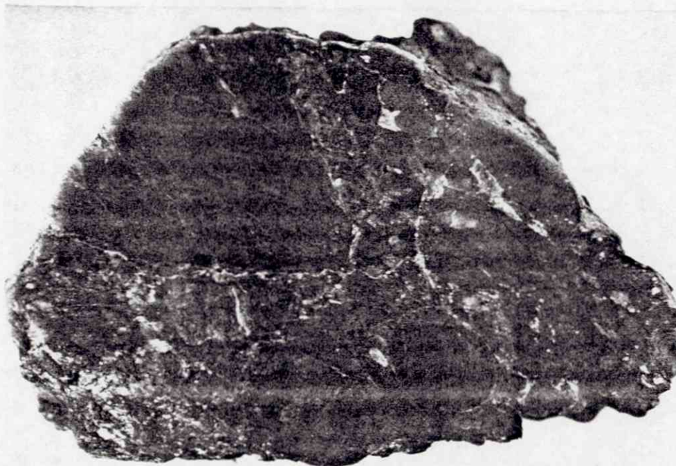
Fig. 43. Prøve nr. 164c.
