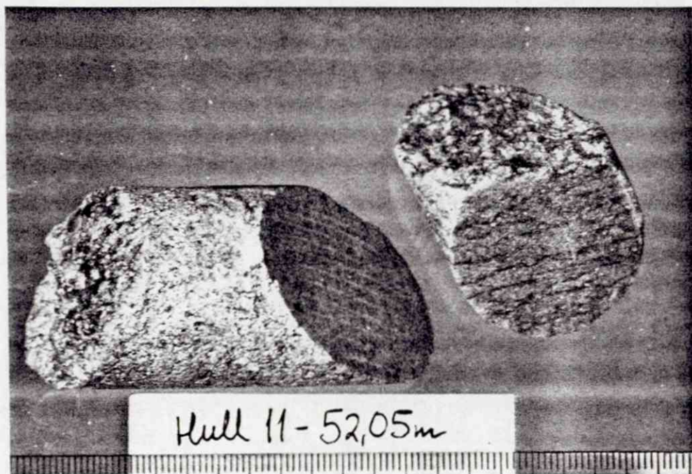
Fig. 36. Kjerneprøve hull 11 - 52,05 m.
