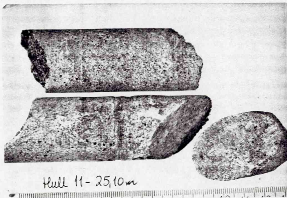
Fig. 27. Kjerneprøve hull 11 - 25,10 m. Omtrentlig mineralfordeling i tilhørende slip: 70-80 % talk, ~ 10 % karbonat, 5-10 % (?) kloritt og ~ 5 % sekundær magnetitt + kromitt. Jfr. mikrosondeanalyse nr. 1 - 7 i Bilag 3, side 1 og 2.
