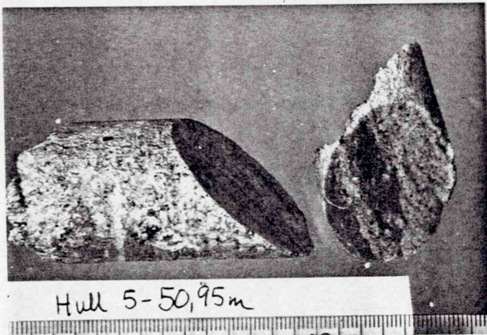
Fig. 10. Kjerneprøve hull 5 - 50,95 m. Omtrentlig mineralfordeling i tilhørende slip: 40-50 % karbonat, 40-50 % talk, ~ 5 % (?) kloritt og ~ 5 % sekundær magnetitt + kromitt. Karbonatene opptrer å samme måte som i fig. 5 - 9. Videre er observert talk pluss finkornet dolomitt og grovkornet breunneritt i aggregatform (mer sammenvokst enn vanlig?).
