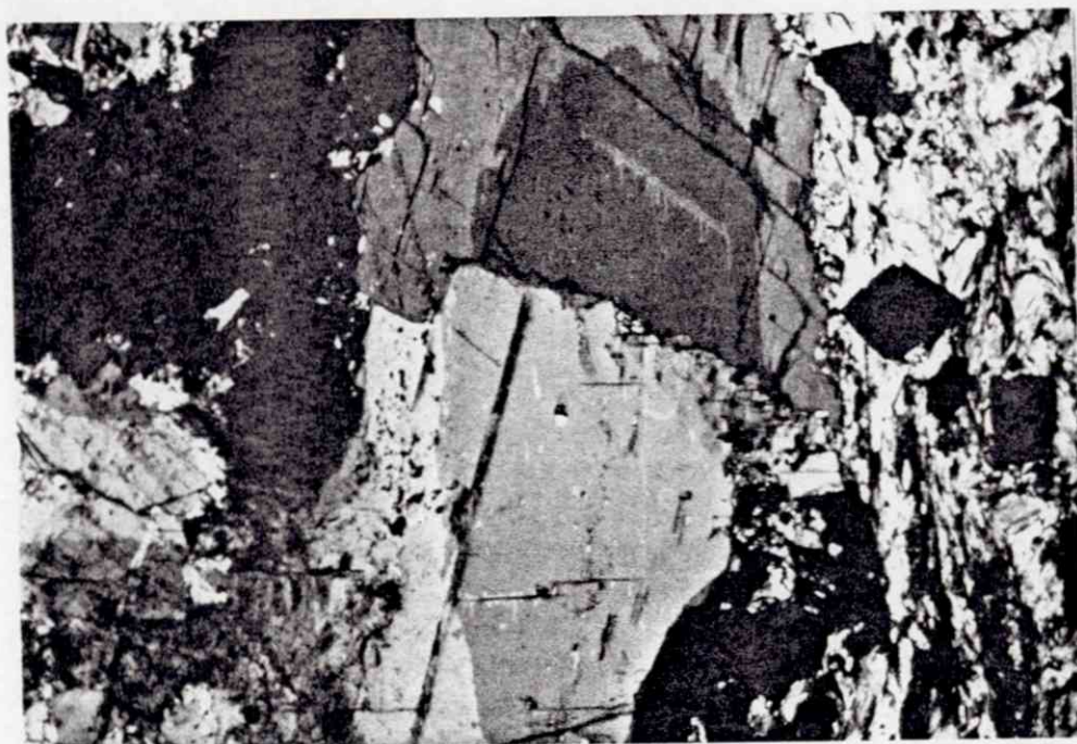
Fig. 6. Mikrofoto av slip 5 - 48,85/område 1.
