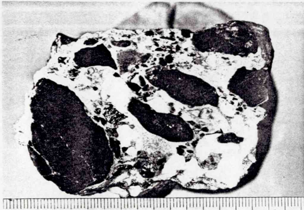
Fig. 46. Prøve nr. 172c.
