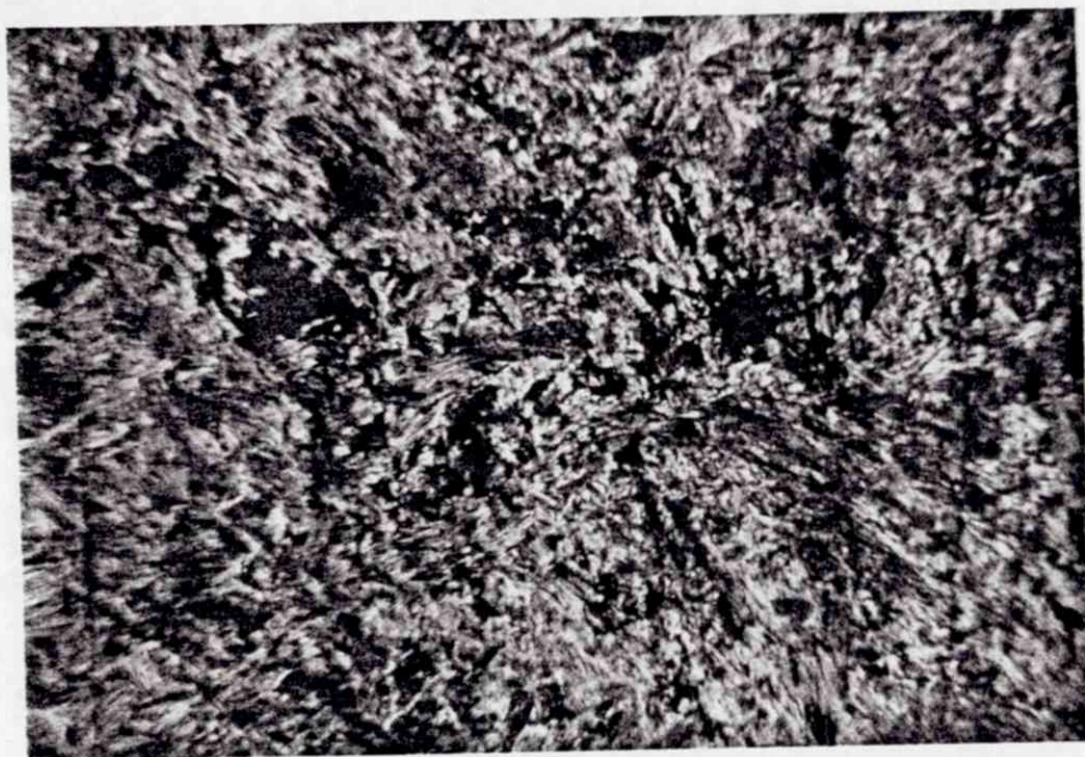
Fig. 14. Mikrofoto av slip 5 - 79,95 m. 12 x forstørrelse og parallelt lys. Små partier av kloritt (brunsvart) intimt sammenvokst med talk (fra lys brun til gulhvitt). To små oksydkorn (svarte) sentralt på bildet.
