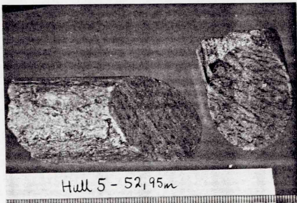
Fig. 11. Kjerneprøve hull 5 - 52,95 m. Omtrentlig mineralfordeling i tilhørende slip: ~ 60 % karbonat, ~ 30 % talk, <5 % (?) kloritt og ~ 5 % sekundær magnetitt + kromitt.
