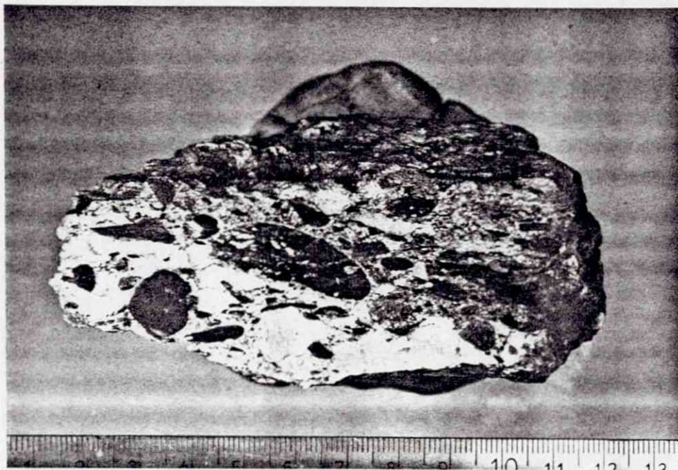
Fig. 42. Prøve nr. 133a.
