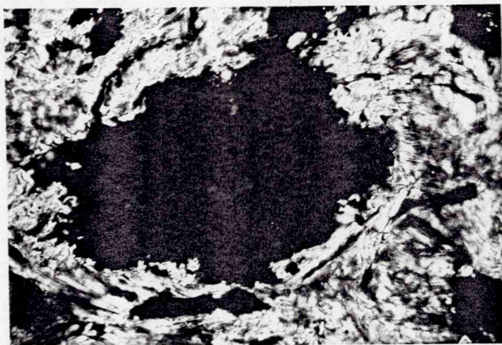
Fig. 28. Mikrofoto av slip 11 - 25,10 m/område 2. 160 x forstørrelse, kryssede nicols. Et ørlite klorittkorn (merk forstørrelsen) med anomal mørkebrun og -berlineblå interferensfarve. Ofte er slike brune partier noe mer Mg-dominert enn de blå partiene, mens de blå til gjengjeld er noe sterkere Fe-dominert. Slike tendenser kunne imidlertid ikke spores ved mikrosondeanalyser innenfor kornet. Se analyse 1 - 4 i Bilag 3, side 1.
