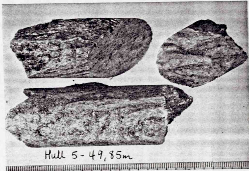
Fig. 9. Kjerneprøve hull 5 - 49,85 m. Omtrentlig mineralfordeling i tilhørende slip: ~ 70 % karbonat, 25-30 % talk og ~ 5 % sekundær magnetitt pluss kromitt. Karbonatopptreden på samme måte som i fig. 5 - 8.
