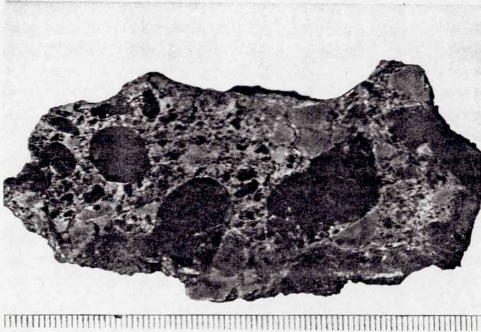
Fig. 45. Prøve nr. 170b.
