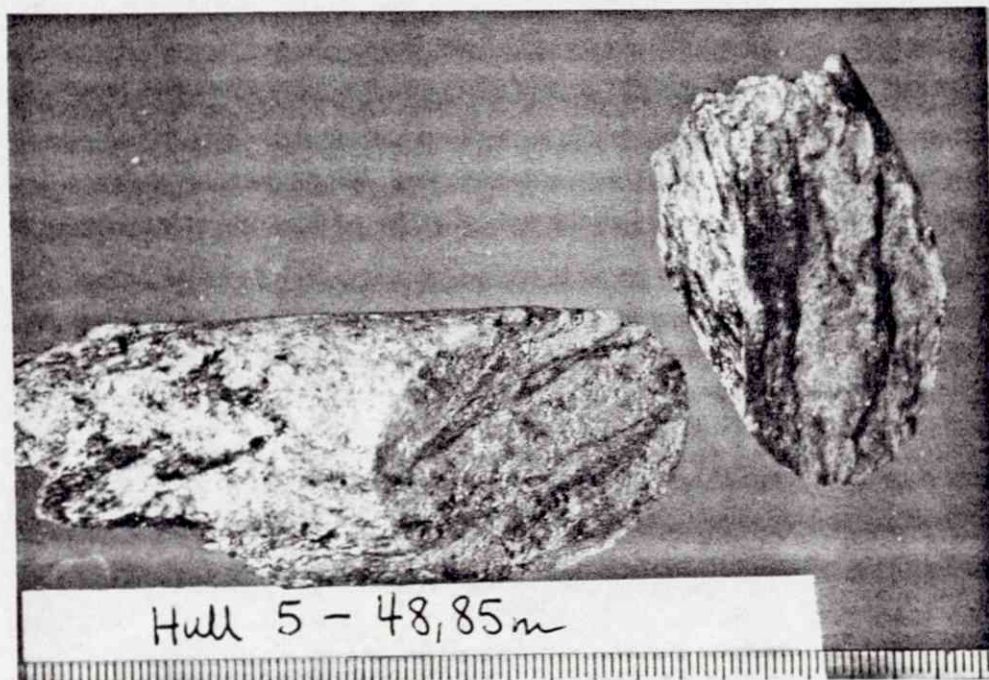
Fig. 5. Kjerneprøve hull 5 - 48,85 m.
