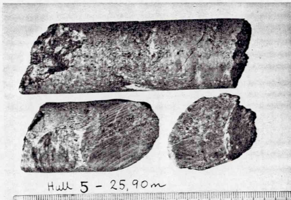
Fig. 3. Kjerneprøve hull 5 - 25,9 m. Omtrentlig mineralfordeling i tilhørende slip: ~ 20 % karbonat, 5-10 % (?) kloritt, et meget finkornet aggregat av ~ 50 % talk og ~ 25 % serpentinerester og tilslutt ~ 5 % kromitt og sekundær magnetitt. I slipet kan sees serpentin under omvandling til talk både i boller og matriks. Enkelte små serpentin"boller" (egentlig sandkorn og gruskorn av serpentin) er helt uangrepet av talkifiseringsprosessen.
