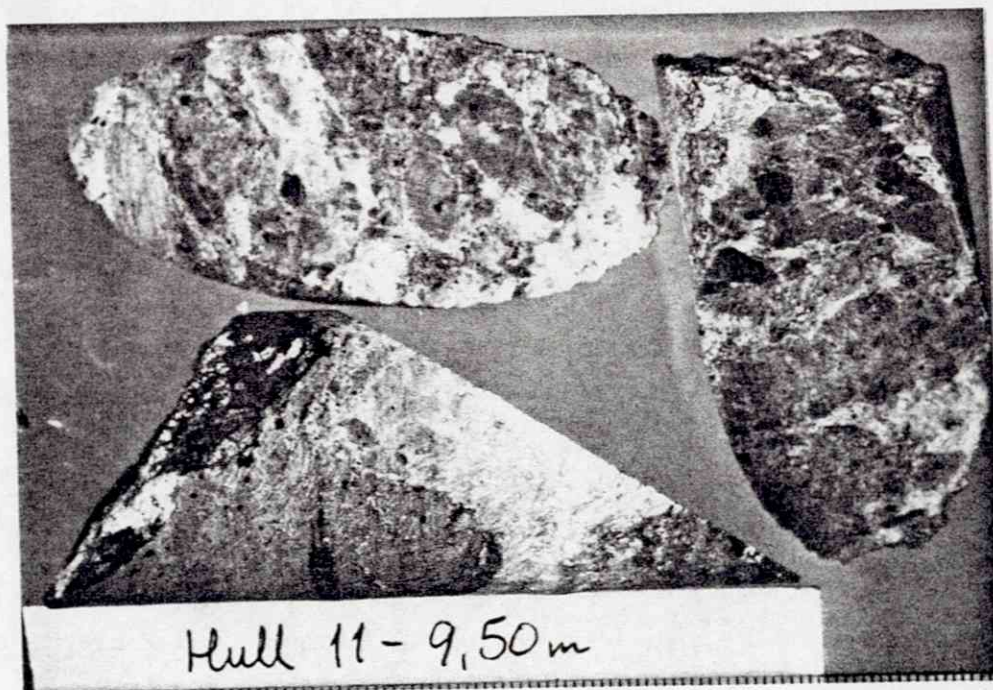
Fig. 22. Kjerneprøve hull 11 - 9,50 m. Omtrentlig mineralfordeling i tilhørende slip: 40-50 % karbonat, et finkornet aggregat av ~ 40 % talk og ~ 10 % (?) serpentinerester. Videre <5 % kloritt og 3-4 % sekundær magnetitt pluss kromitt. Prøven viser noe sterkere omvandling enn prøve 11 - 8,20 m.
