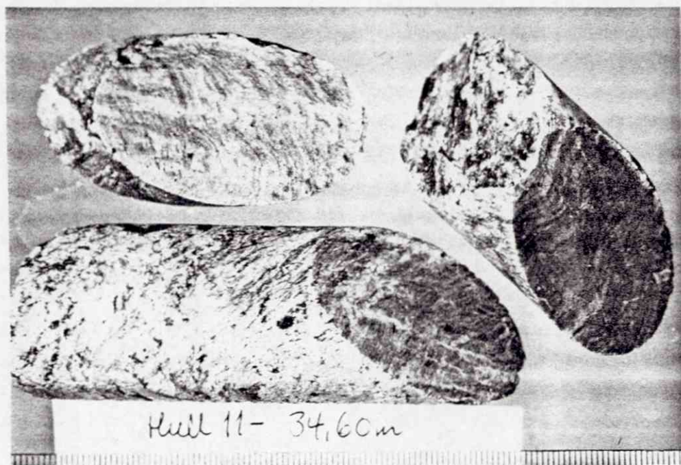
Fig. 32. Kjerneprøve hull 11 - 34,60 m.
