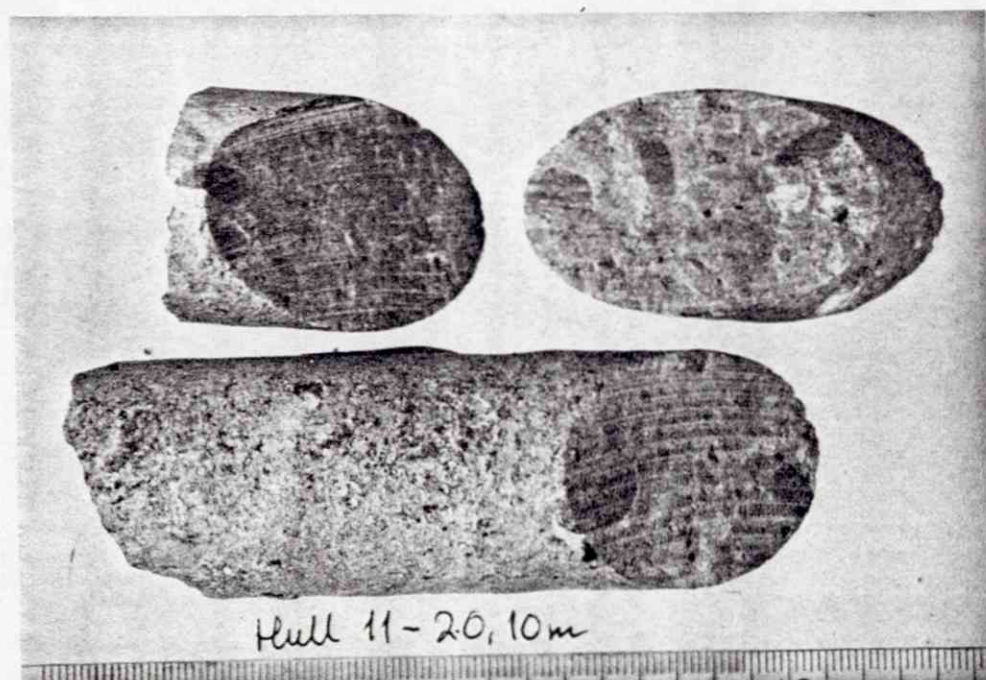
Fig. 26. Kjernprøve hull 11 - 20,10 m. Omtrentlig mineralfordeling i tilhørende slip: 60-70 % talk, 20-30 % serpentinrester, ~ 5 % kloritt og ~ 5 % sekundær magnetitt pluss kromitt. Jfr. mikrosondeanalyse nr. 10 og 11 i Bilag 3, side 3.
