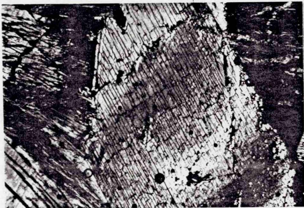
Fig. 17. Mikrofoto av slip 5 - 81,75 m/område 3. 25 x forstørrelse og kryssede nicols. Aktinolittnåler (med flere farver) i en kloritt grunnmasse (mørk grønn). Jfr. mikrosondeanalyse nr. 16, Bilag 3, side 4.
