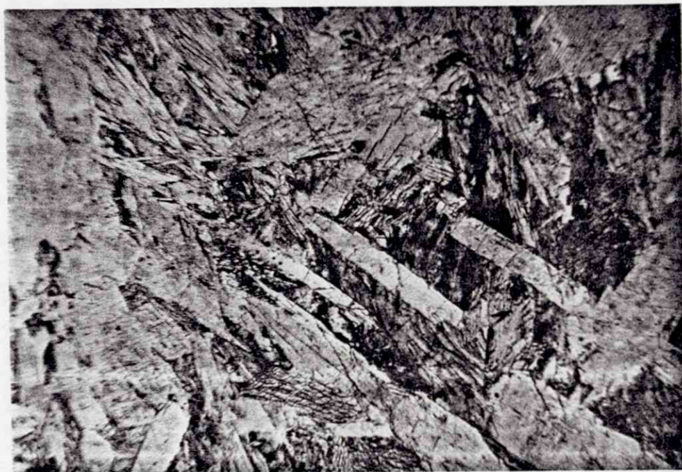
Fig. 19. Mikrofoto av slip 5 - 81,75 m. 6 x forstørrelse og parallelt lys.
