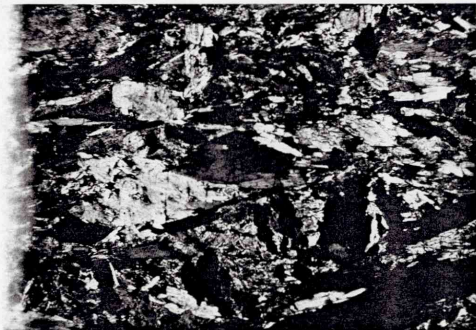
Fig. 37. Mikrofoto av slip 308 B fra Råsdaalsfjell.
