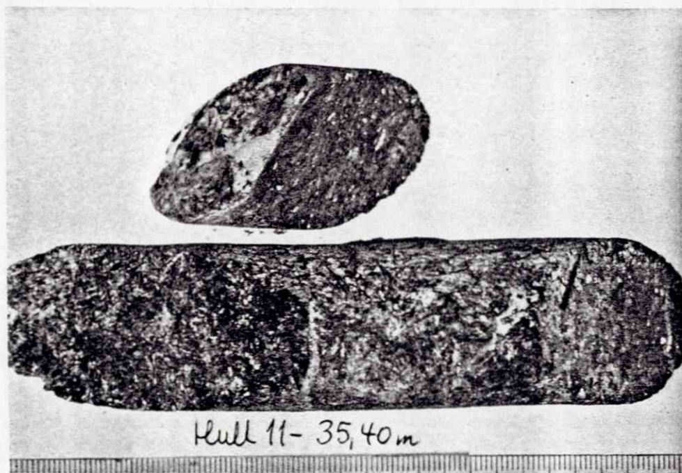
Fig. 33. Kjerneprøve hull 11 - 35,40 m.
