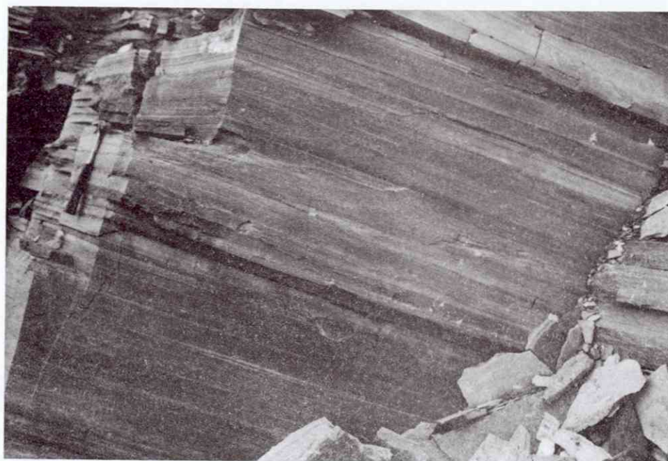
Fig. 3. Tverrsnitt av samme benk som vist på fig. 2. (dvs. snittflaten vinkelrett på strøkretingen). Her vises foldene og uregelmessighetene tydelig. Foto tatt i lokalitet nr. 6.
