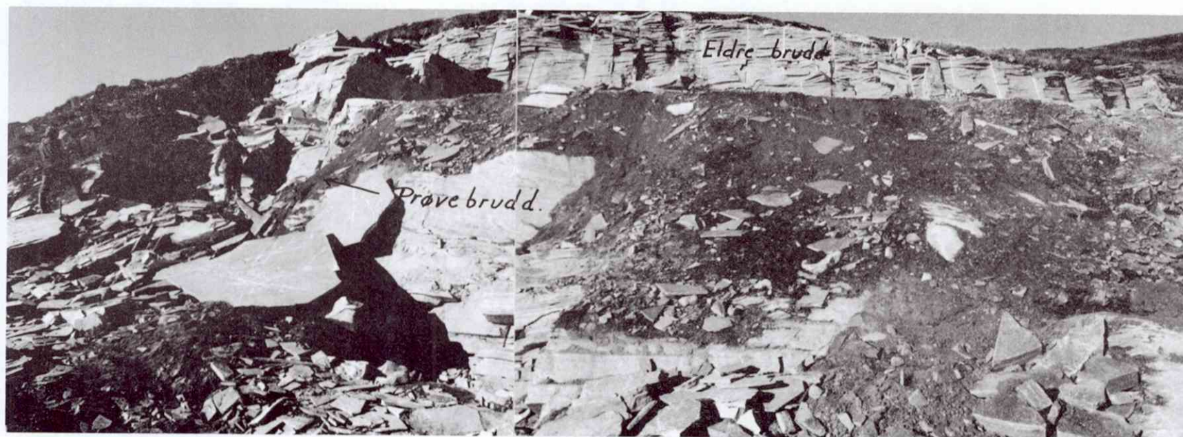
Fig. 6. Bruddområde 1 med skiferlag 1, sett fra anleggsveien og oppover (nordover).
