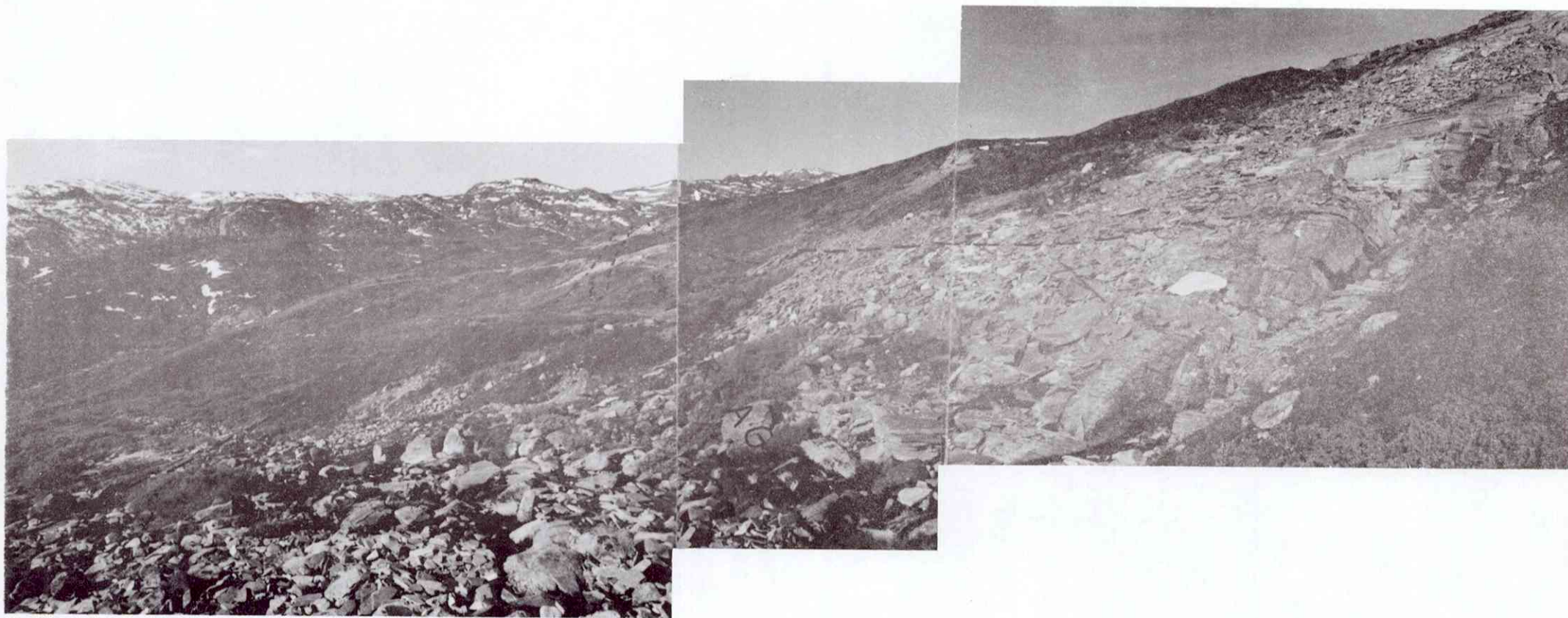
Fig. 7. Skiferlag 1 i bekken ved bruddområde 2. Sett vestover mot bruddområde 1. Kløften sees til høyre i bildet.
