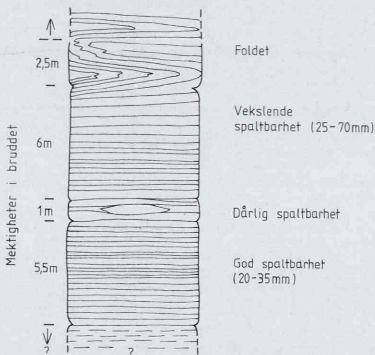
Fig.1 Skjematisk fremstilling av forholdene i bruddomr. 1.
