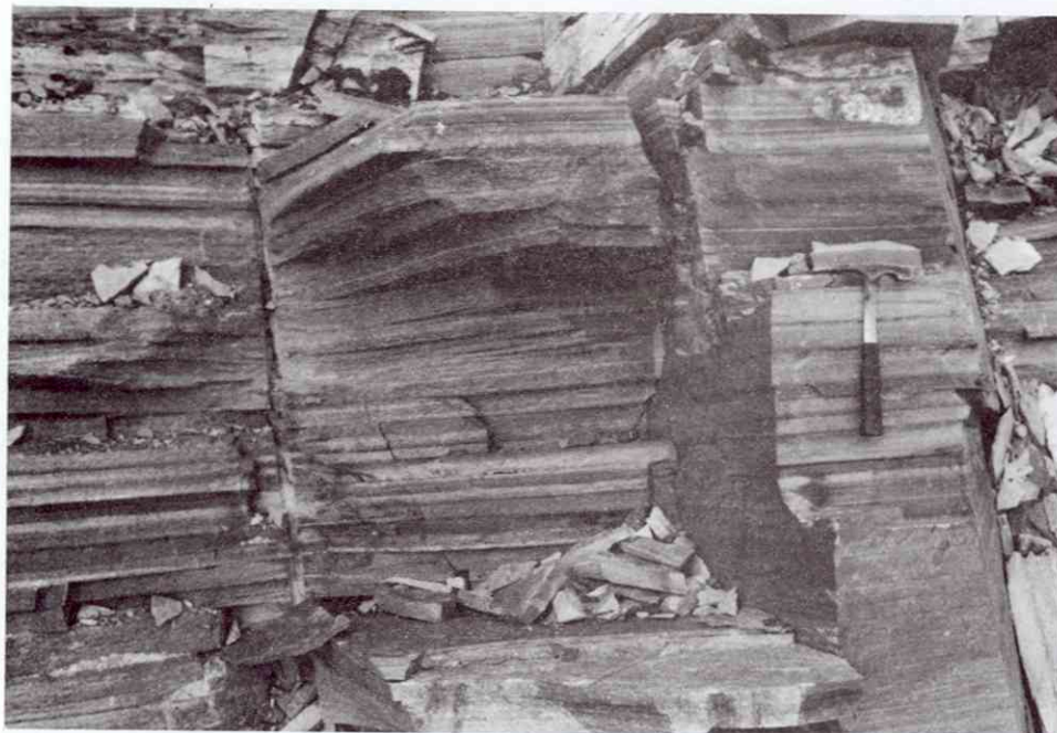
Fig. 2. I bruddfronten (dvs. snittflaten parallelt strøkretingen) vises ikke foldene så tydelig.
