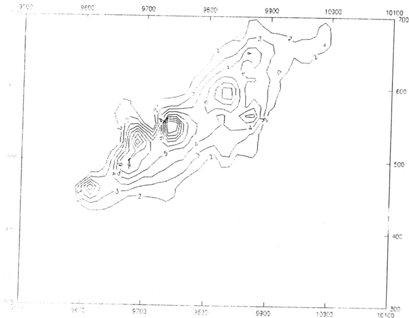
FIG. 4 ISOPACH-KART ZN-GEHALT
