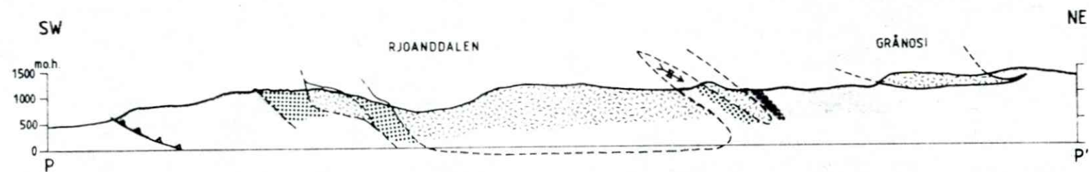
Fig. 4. Profil P-P' (se bil. 06) gjennom sydvestlige deler av Jotundekket ved Mjølfjell. Tegnforklaring som for fig. 1.
