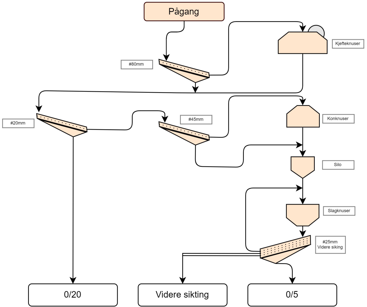
Vedlegg 3 - Optimalisert flytskjema
