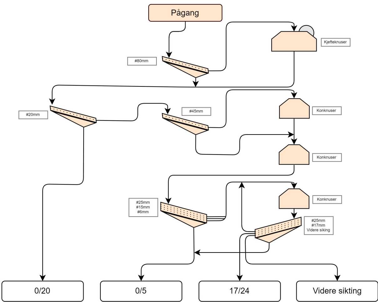
Vedlegg 3 - Optimalisert flytskjema
